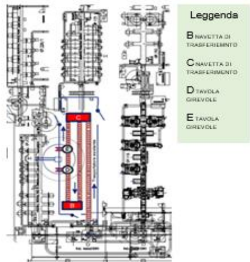
Nuovo Lay-out indicativo futuro con 2 navette
