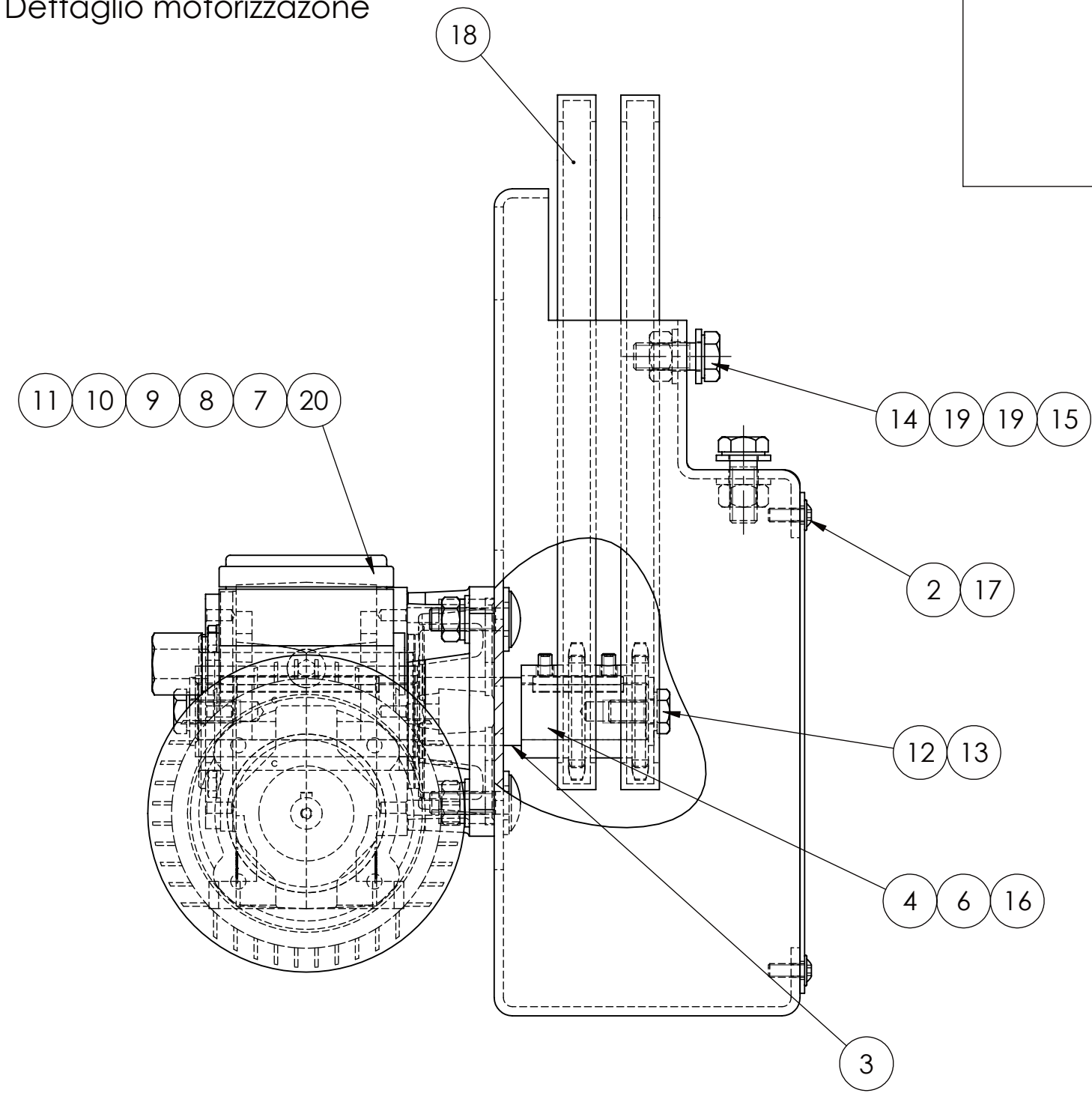
1RU03-1200-0058 Dettaglio motorizzazione
