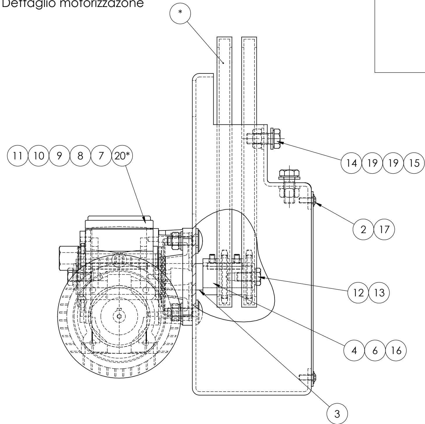
1RU03-1200-0058_001 Dettaglio motorizzazione
