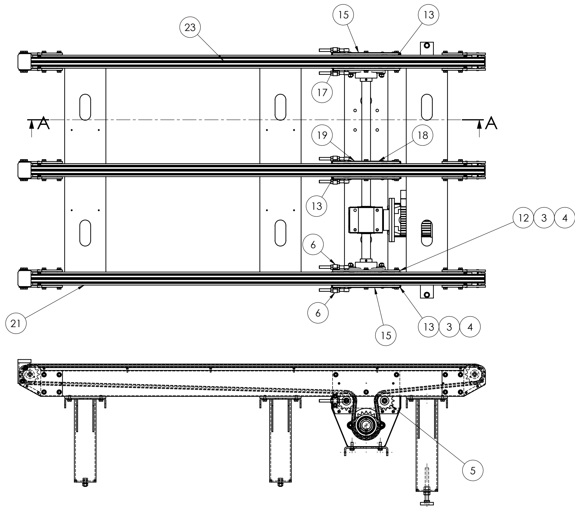
SEZIONE A-A
