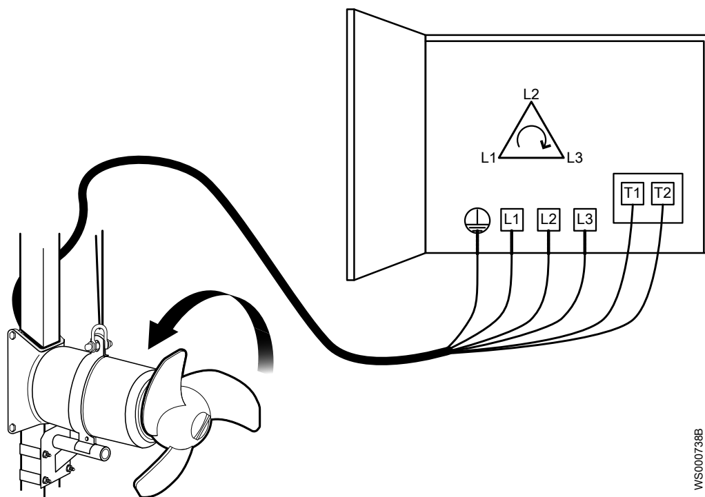
Afbeelding 8: Juiste motorkabelverbinding
