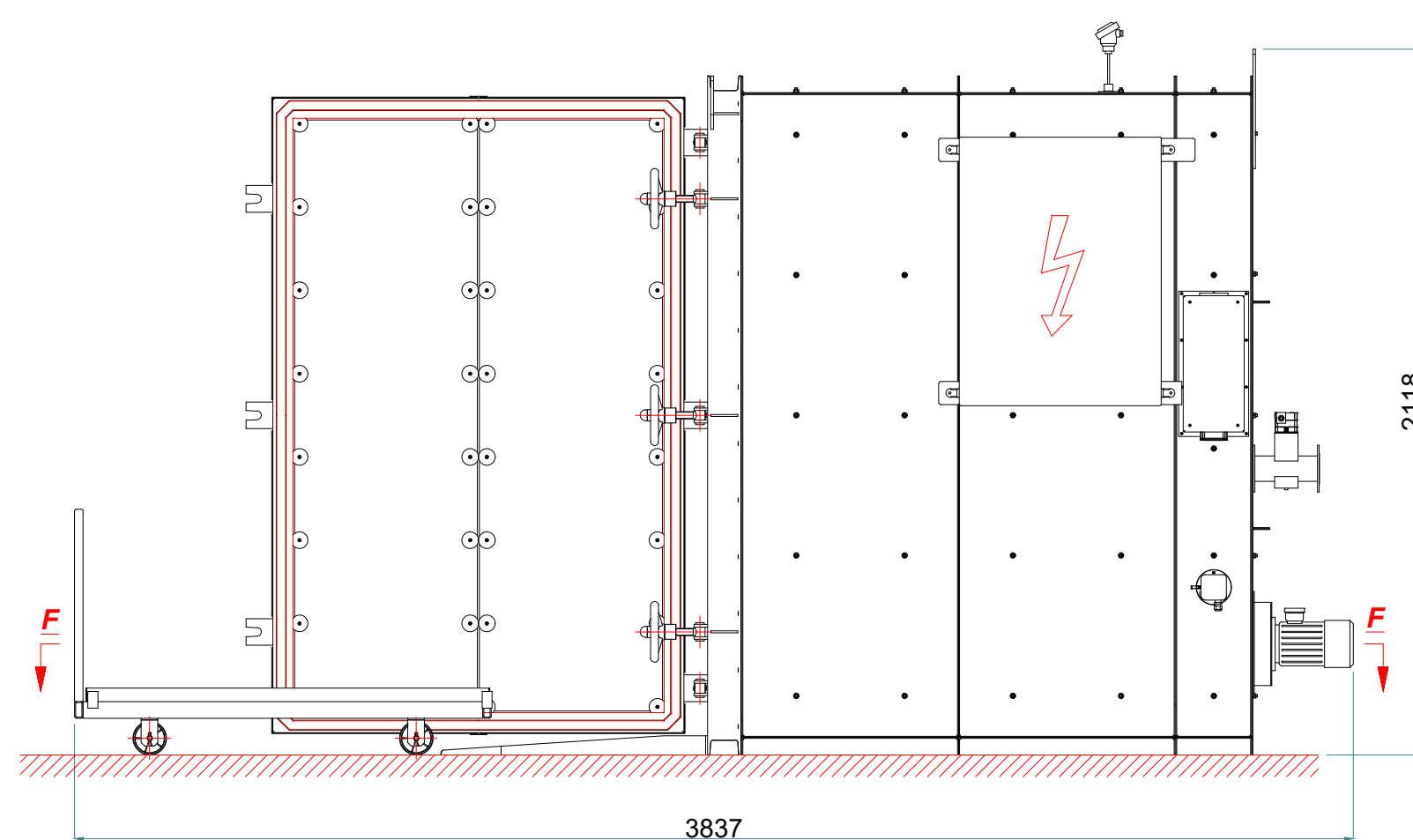
PROSPETTO CON CARRELLO ESTRATTO ( 1 : 20 )
