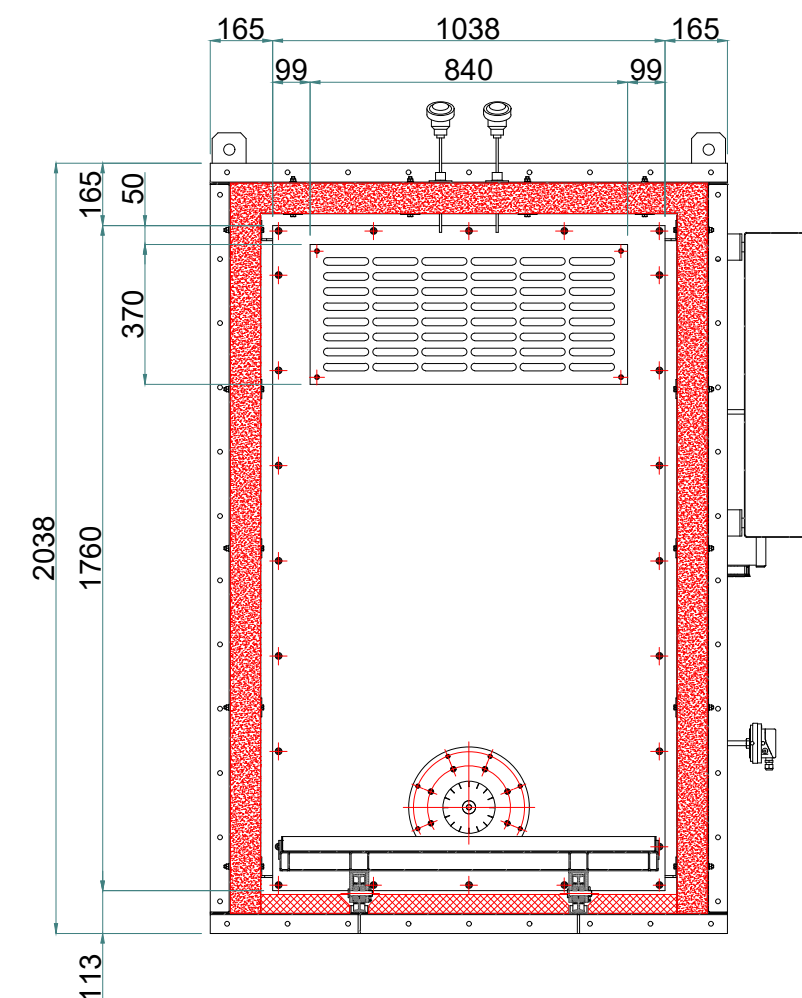
C-C ( 1 : 20 )
