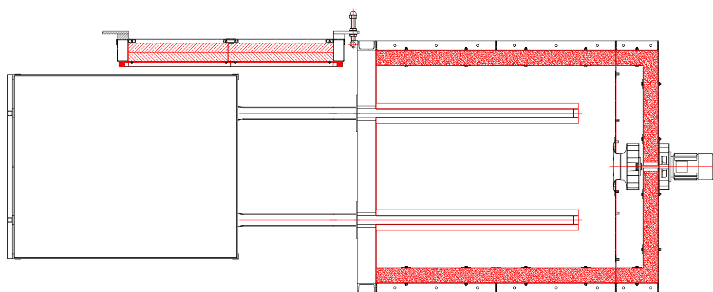
F-F ( 1 : 20 ) PIANTA CON CARRELLO ESTRATTO
