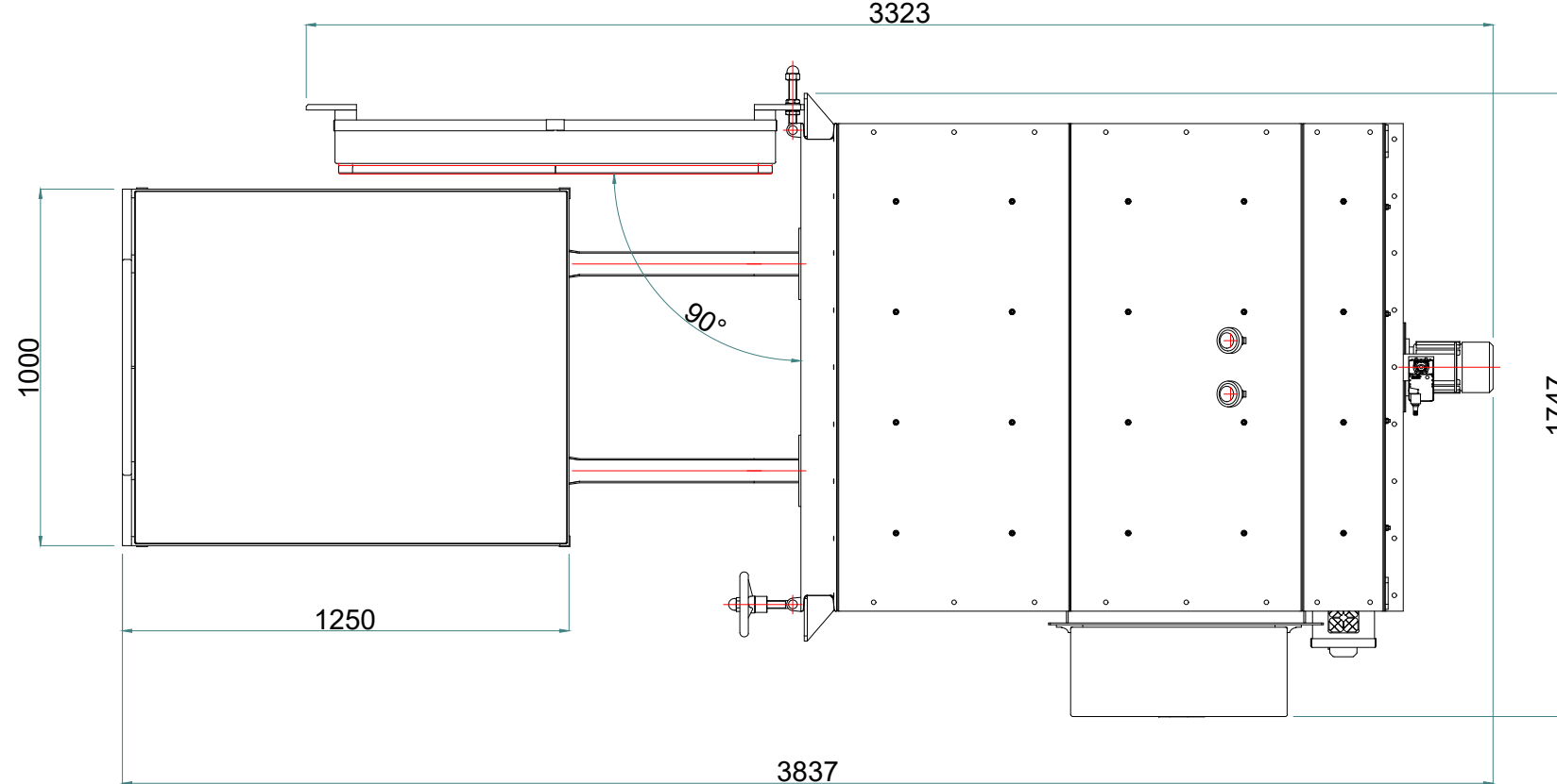
PIANTA CON CARRELLO ESTRATTO ( 1 : 20 )
