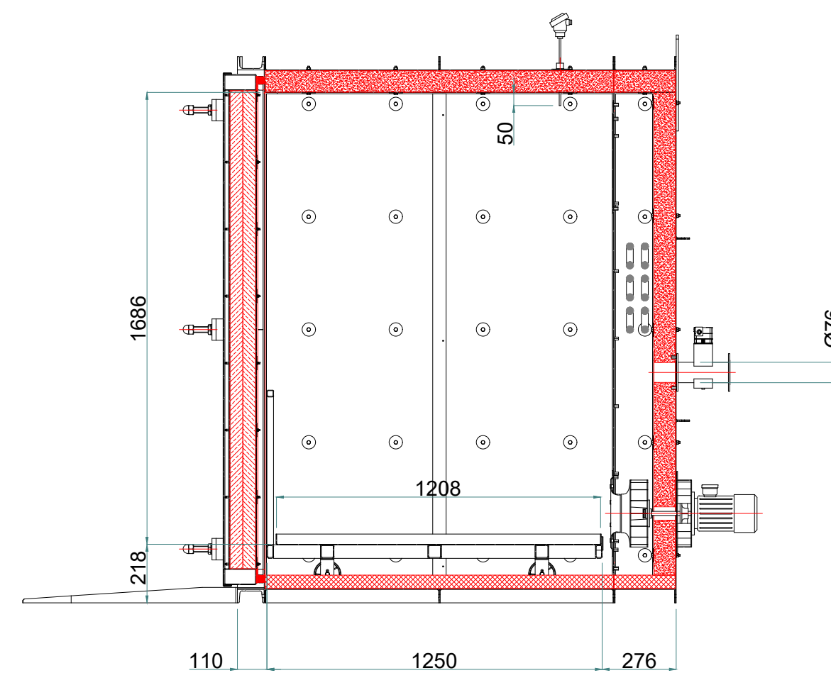
A-A ( 1 : 20 )
