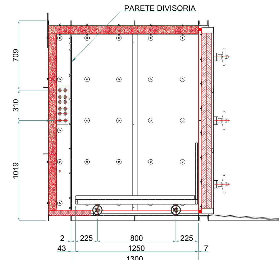
B-B ( 1 : 20 )
