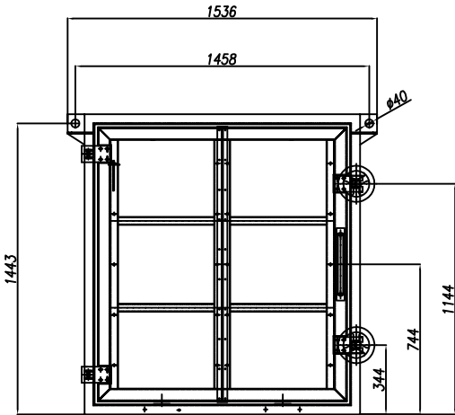
Vista da "A" Dettaglio Porta
