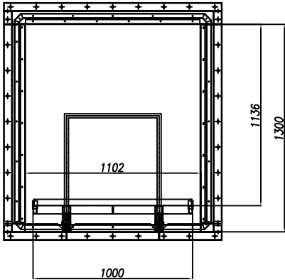
Vista da "A" Dettaglio Porta
