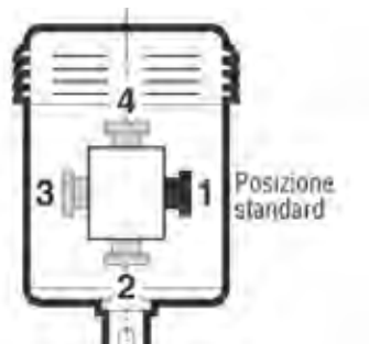
Posizioni del pressacavo rispetto all'estremità d'albero motore
