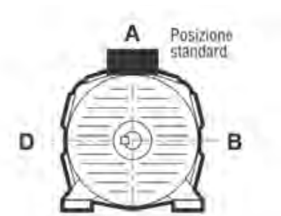
POSIZIONE SCATOLA MORSETTIERA E POSIZIONE USCITA CAVI
