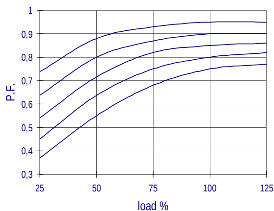
\cos\phi - POWER FACTOR - LEISTUNGSFAKTOR BEI VOLLAST
