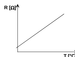
PT 100
