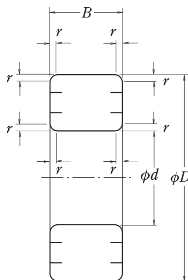
Fig. 7.1 Dimensioni di ingombro dei cuscinetti radiali
