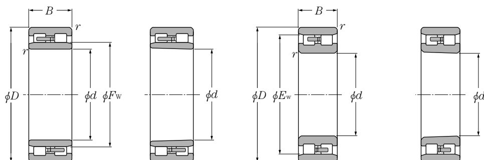
Tipo NNU Foro cilindrico Foro conico conicità 1:12 Tipo NN Foro cilindrico Foro conico conicità 1:12
