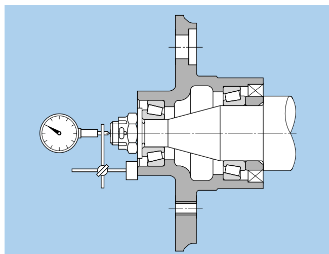
Fig. 15.13 Misurazione della registrazione del gioco assiale
