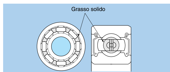
Fig. 11.3 Cuscinetto radiale a sfere con grasso solido "Spot-pack" (Schermi Z) (Standard per i cuscinetti radiali a sfere)
