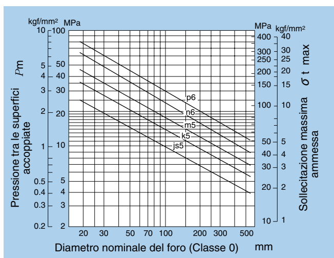
Fig. 17.5.2 Accoppiamento con interferenza massima, pressione superficiale massima p m e sollecitazione ammissa σ t max
