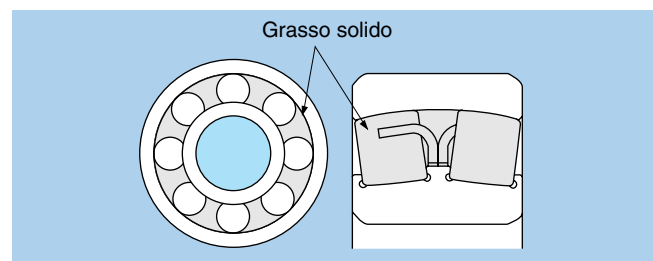
Fig. 11.4 Cuscinetto orientabile a rulli con grasso solido "Full-pack" (Standard per i cuscinetti orientabili a rulli)
