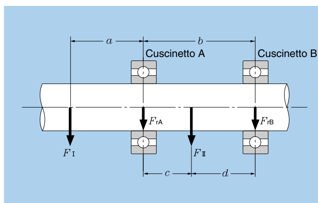
Fig. 4.7 Gruppo albero ingranaggi
