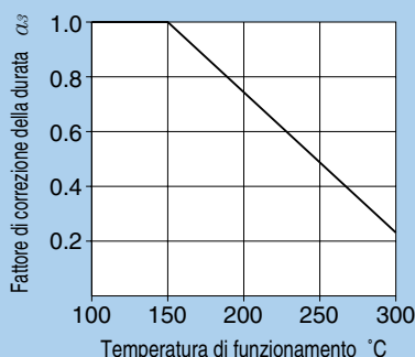
Fig. 3.2 Fattore correttivo della durata relativo alle condizioni operative
