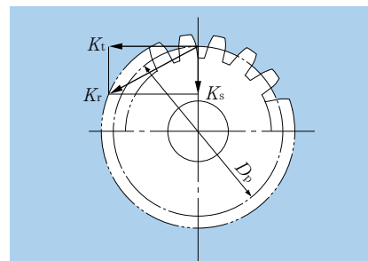
Fig. 4.3 Forza radiale risultante
