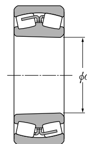
Foro conico conicità 1:12 (K) 1:30 (K30)
