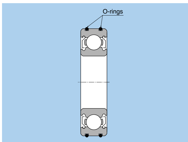
Fig.3 Cuscinetto AC
