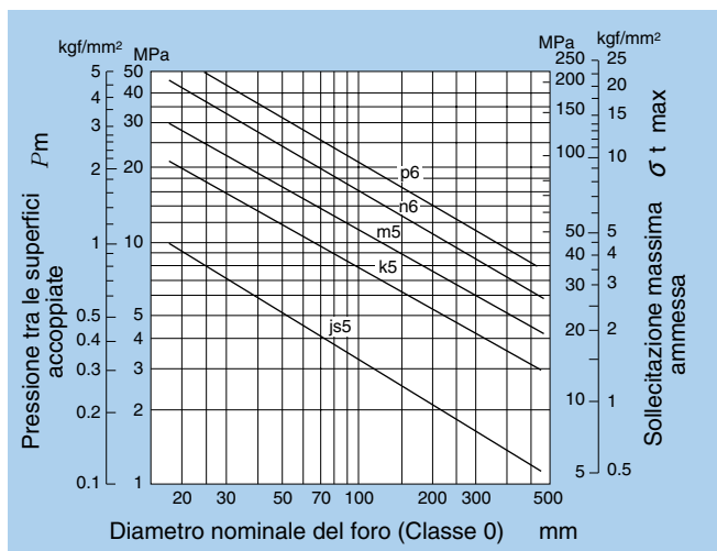
Fig. 17.5.1 Accoppiamento con interferenza media, pressione superficiale massima p m e sollecitazione ammissa σ t max
