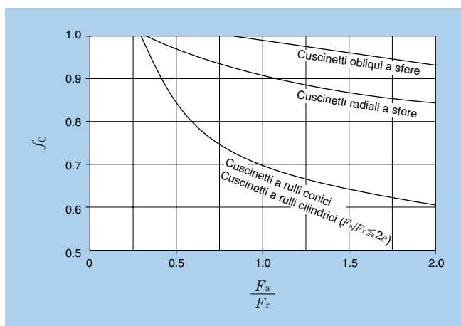
Fig. 9.2 Valore del fattore correttivo f_C dipendente da un carico combinato
