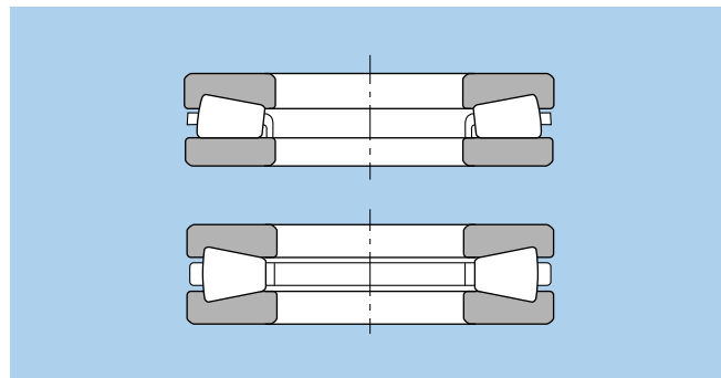
Fig.4 Cuscinetti assiali a rulli conici
