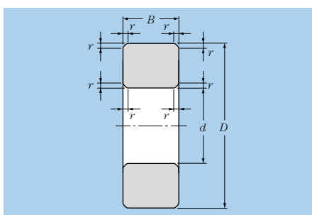
Fig. 5.1 Cuscinetti radiali (esclusi i cuscinetti a rulli conici)
