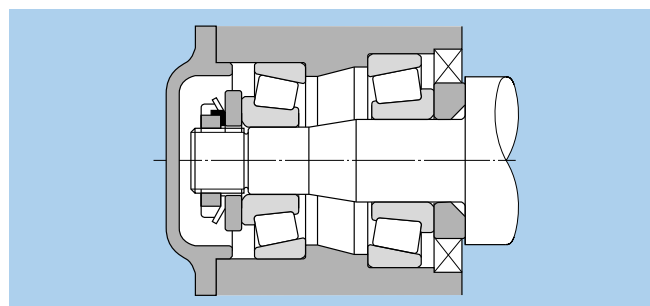
Fig. 15.12 Registrazione del gioco assiale
