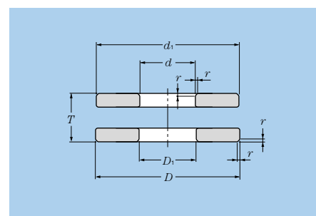
Fig. 5.3 Cuscinetto assiale a semplice effetto
