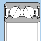
Tipo con tenute non a contatto (LLM)
