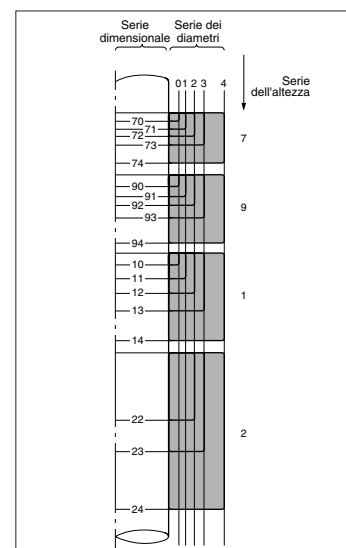
Fig. 5.6 Serie dimensionali dei cuscinetti assiali
