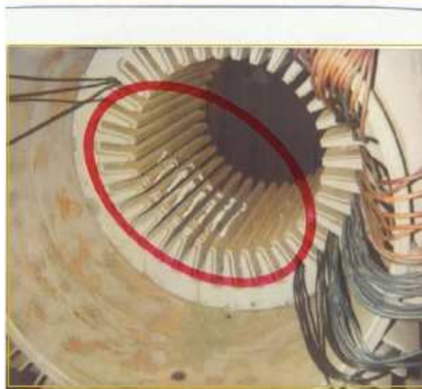
Fase di Collaudo Pacco lamellare Motore A mezzo Termo-grafia a Raggi Infrarossi – RING-TEST
