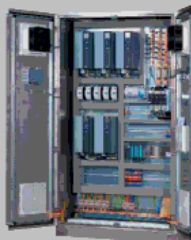
Quadro inox comando e controllo n.5 pompe da 18.5 kW
