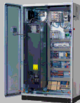
Quadro di comando e controllo idro-generatore da 100 kW
