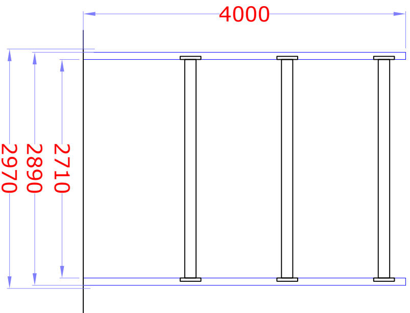
Prospetto frontale
