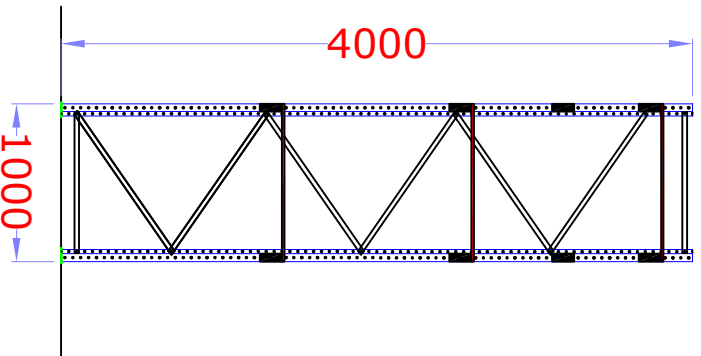
Prospetto laterale
