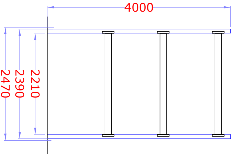
Prospetto frontale
