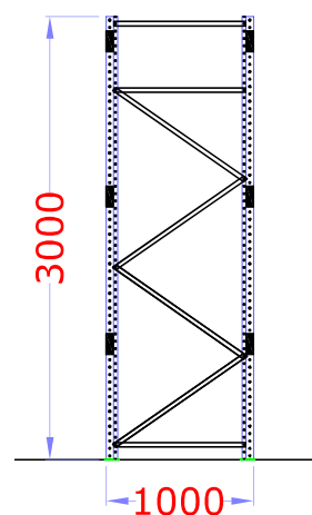
Prospetto laterale
