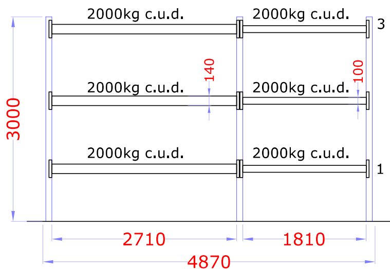
Prospetto frontale
