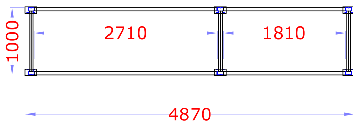
Pianta
