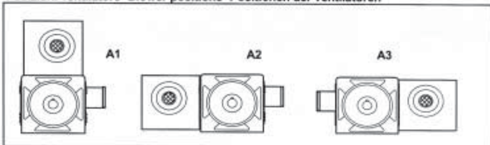
Posizioni ventilatore- Blower positions- Positionen der ventilatoren
