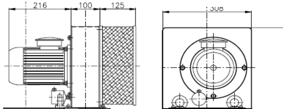
GRUPPO P 160 -Asincr. 0,55Kw 2P 3x230/400V 50Hz
