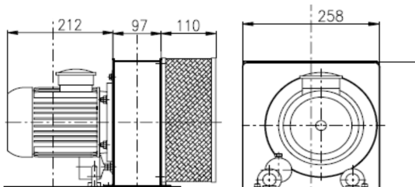
GRUPPO P 132 -Asincr. 0,37Kw 2P 3x230/400V 50Hz
