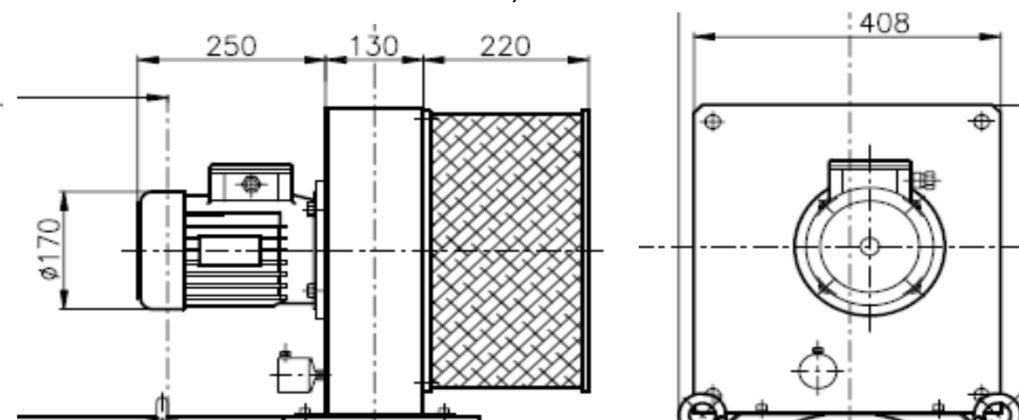
GRUPPO P 200 -Asincr. 2,2Kw 2P 3x230/400V 50Hz
