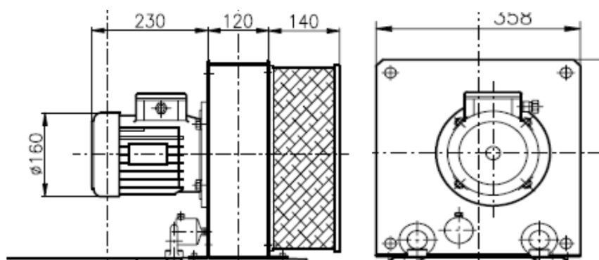
GRUPPO P 180 -Asincr. 1,1Kw 2P 3x230/400V 50Hz
