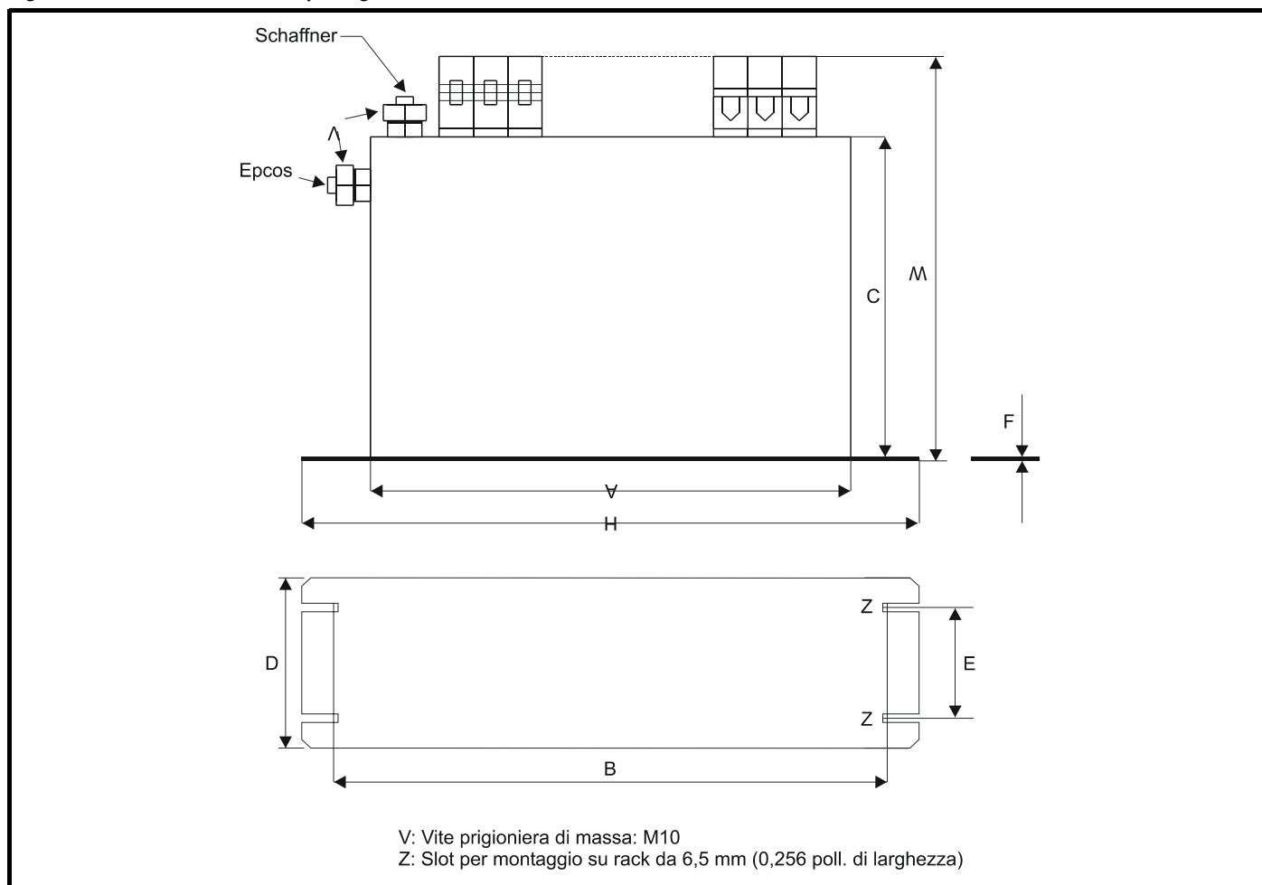
Figura 3-36 Filtro EMC esterno per taglie 4 e 5
