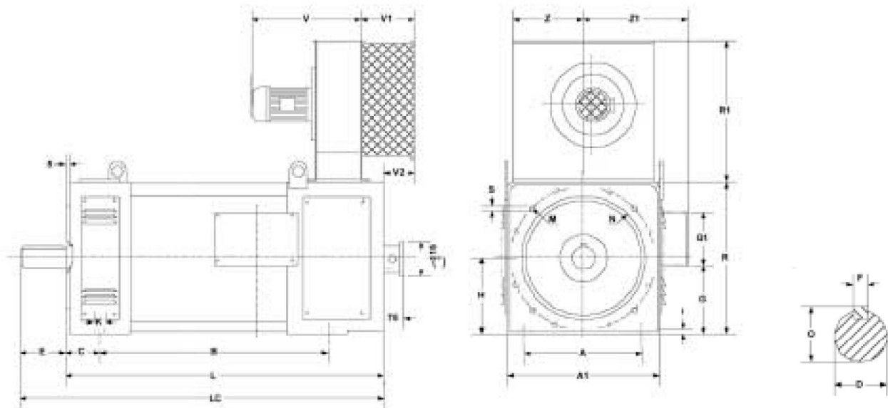
MOTORE CC SERIE LDH VERSIONE IP23 – IC06 – FORMA B3 B5
