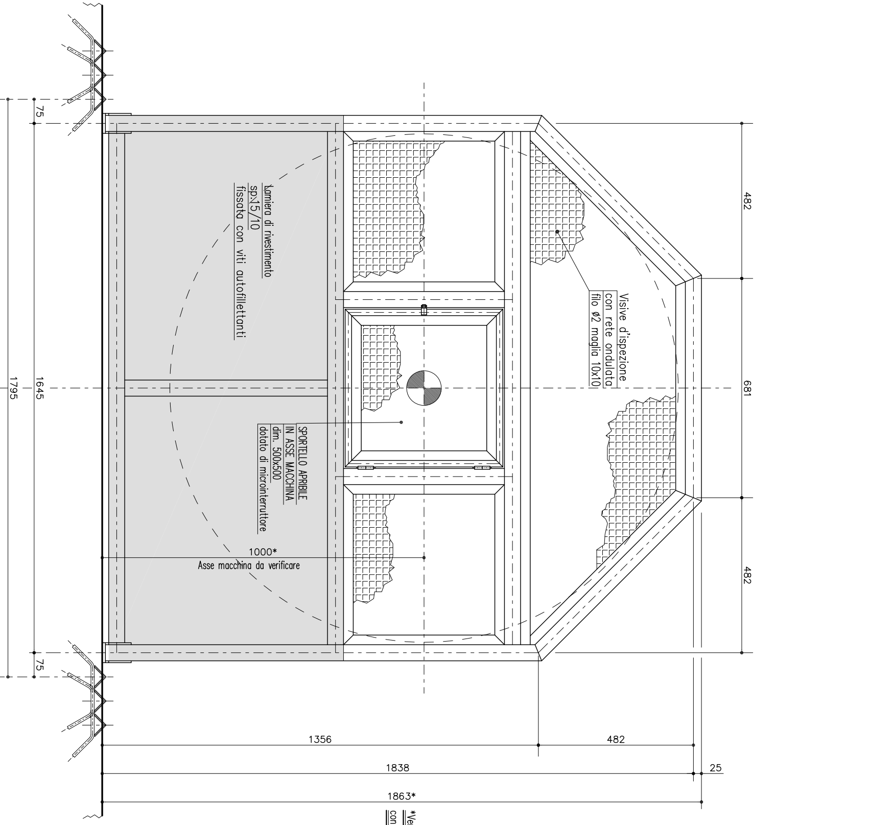
SEZIONE TIPICA C-C CHIUSURA FISSA A PAVIMENTO
