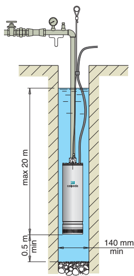
Pompa sospesa
