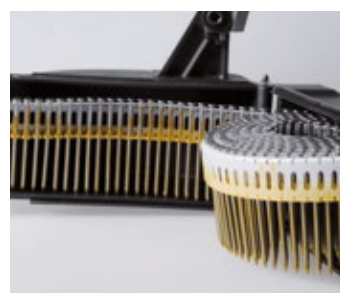
Caricatore chiodi CNP 60
