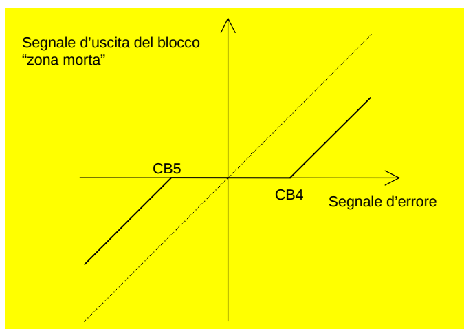
Figura 2C.1 - 3: funzione "zona morta"
