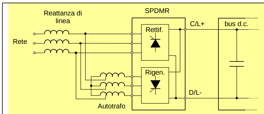
Figura 8A.3 - 1: Schema di collegamento per linee ad alta potenza
