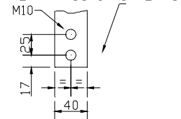
PARTICOLARE ATTACCHI T1-T2-T3
