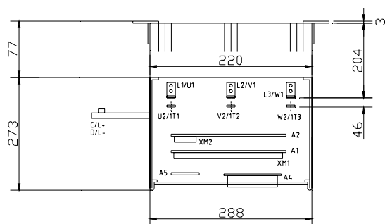
PARTICOLARE ATTACCHI L1-L2-L3
