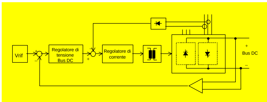
Figura 2C.1 - 1: Schema semplificato del controllo
