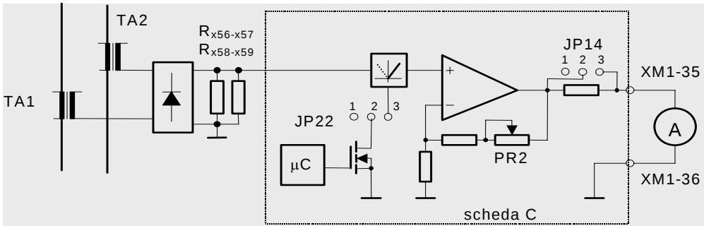
Figura 2C.5 - 1: Schema dell'uscita "la Monitor"
