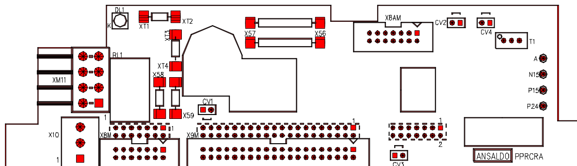
Figura 3.15 - 1: Layout delle schede PPRCRA e PPRCRB
