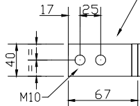
PARTICOLARE ATTACCHI L1-L2-L3
