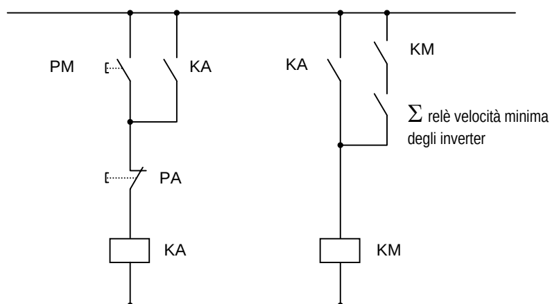
Figura 7A.3 - 3. Esempio di logica di comando
