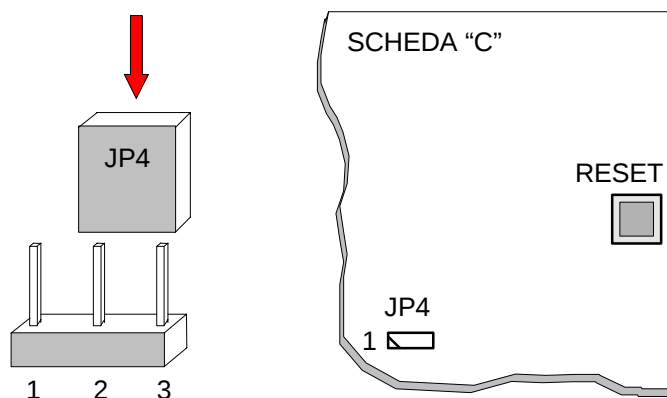
Figura 2C.9.1: Blocco hardware della scrittura dei parametri in EEPROM.
