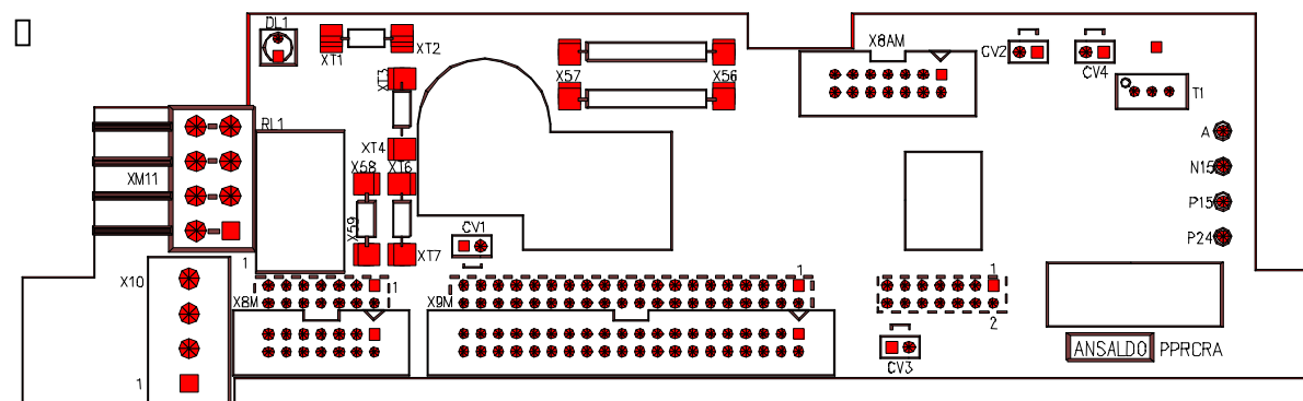
Figura 3.15 - 2: Layout delle schede PPRCRC e PPRCRD
