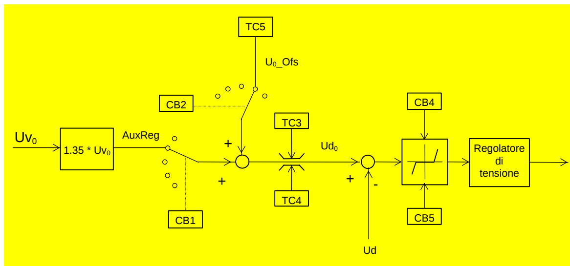
Figura 2C.8 - 1: Offset sul riferimento di tensione d.c.
