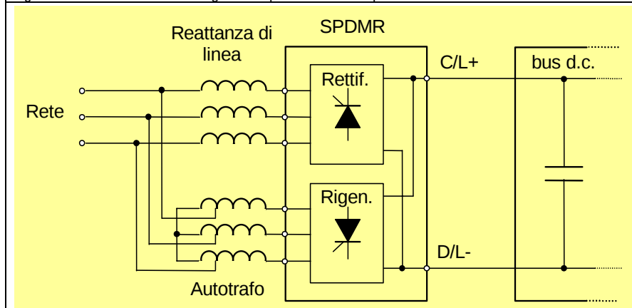
Figura 8A.3 - 2: Schema di collegamento per linee a bassa potenza
