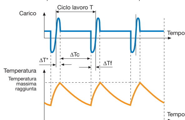
Servizio ininterrotto periodico con frenatura elettrica : Tipo di servizio S7
