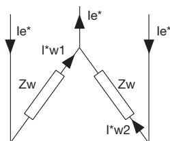
Funzionamento con mancanza di un avvolgimento
