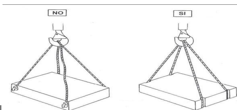
FIG. 3 TIRANTI INCROCIATI
