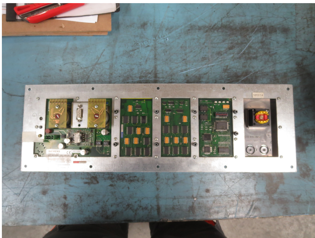
VISTA POSTERIORE TASTIERA
