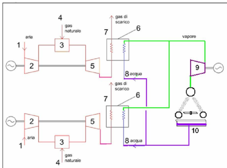
1 Aria comburente; 2 Compressore; 3 Combustore; 4 Gas combustibile; 5 Turbina a gas (espansore); 6 Caldaia a recupero; 7 Scarico fumi al camino; 8 Acqua alimento; 9 Turbina a vapore; 10 Condensatore ad aria forzata.
