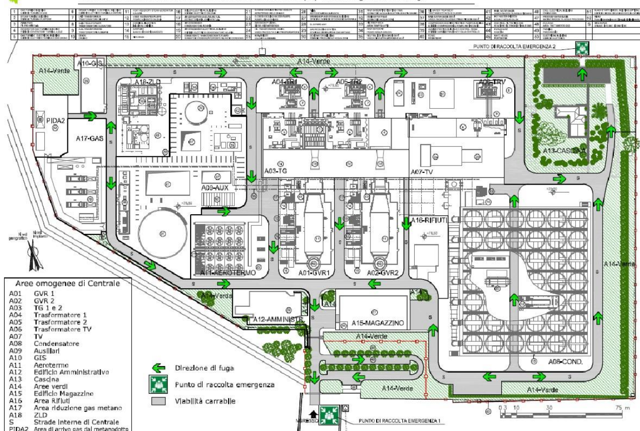
CENTRALE TERMoeLETTRICA A CICLO COMBINATO DI APRILIA (LT) – Aree omogenee e vie di fuga
