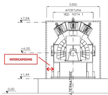
Sez. "E-E"
