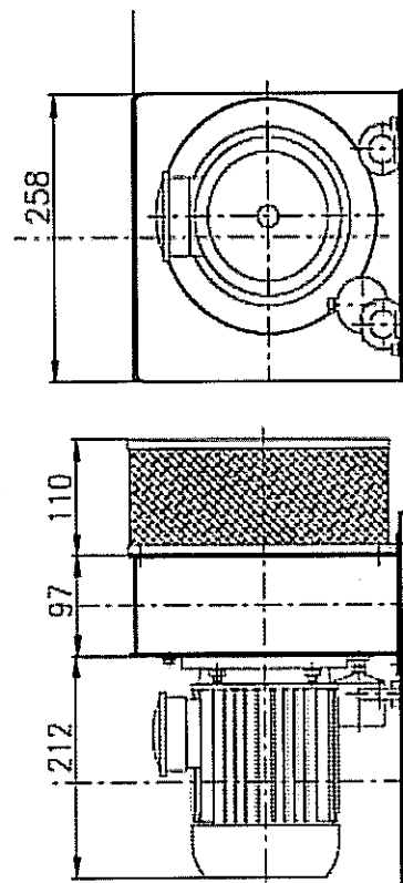
GRUPPO P 132 - Asincr. 0,37Kw 2P 3x230/400V 50Hz
