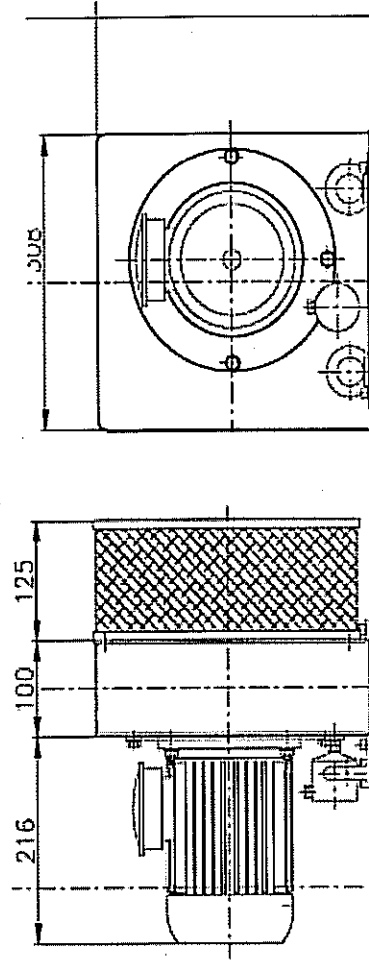
GRUPPO P 160 - Asincr. 0,55Kw 2P 3x230/400V 50Hz
