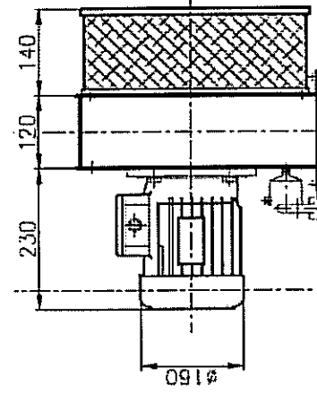
GRUPPO P 180 - Asincr. 1,1Kw 2P 3x230/400V 50Hz
