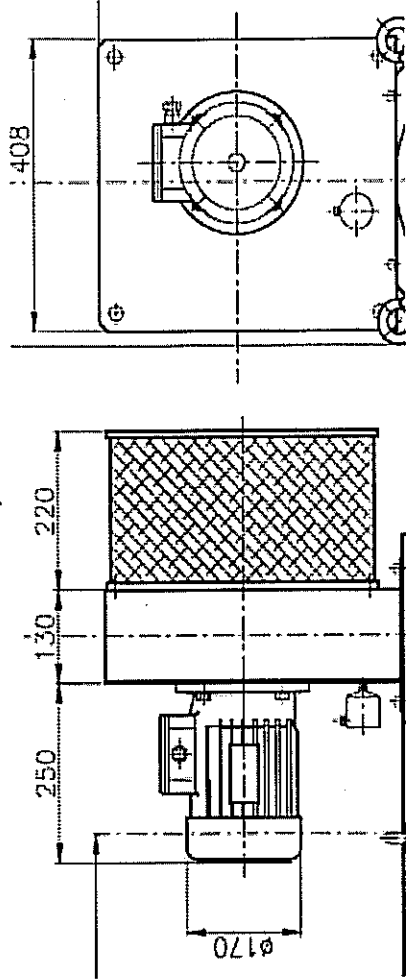
GRUPPO P 200 - Asincr. 2,2Kw 2P 3x230/400V 50Hz
