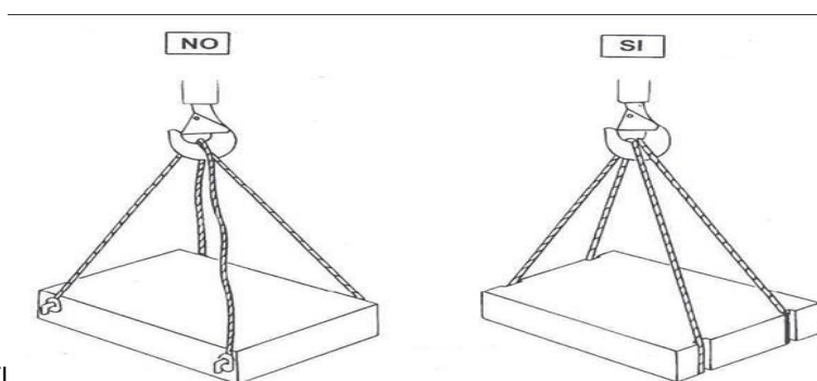
FIG.3 TIRANTI INCROCIATI
