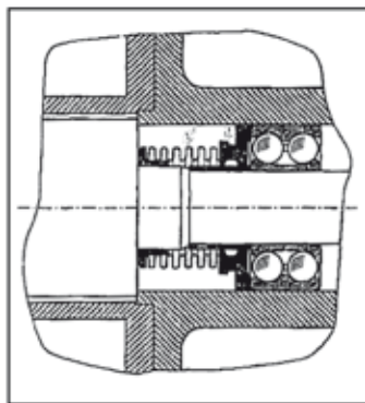
Tipo E Tenuta frontale a soffiello con rasamenti in widia Front bellow seal with Widia shims
