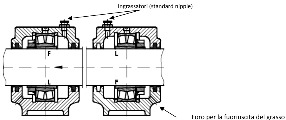
Supporti con cuscinetti a rulli e con bussola di trazione
