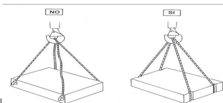
FIG. 3 TIRANTI INCROCIATI
