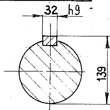
Sezione S-S
