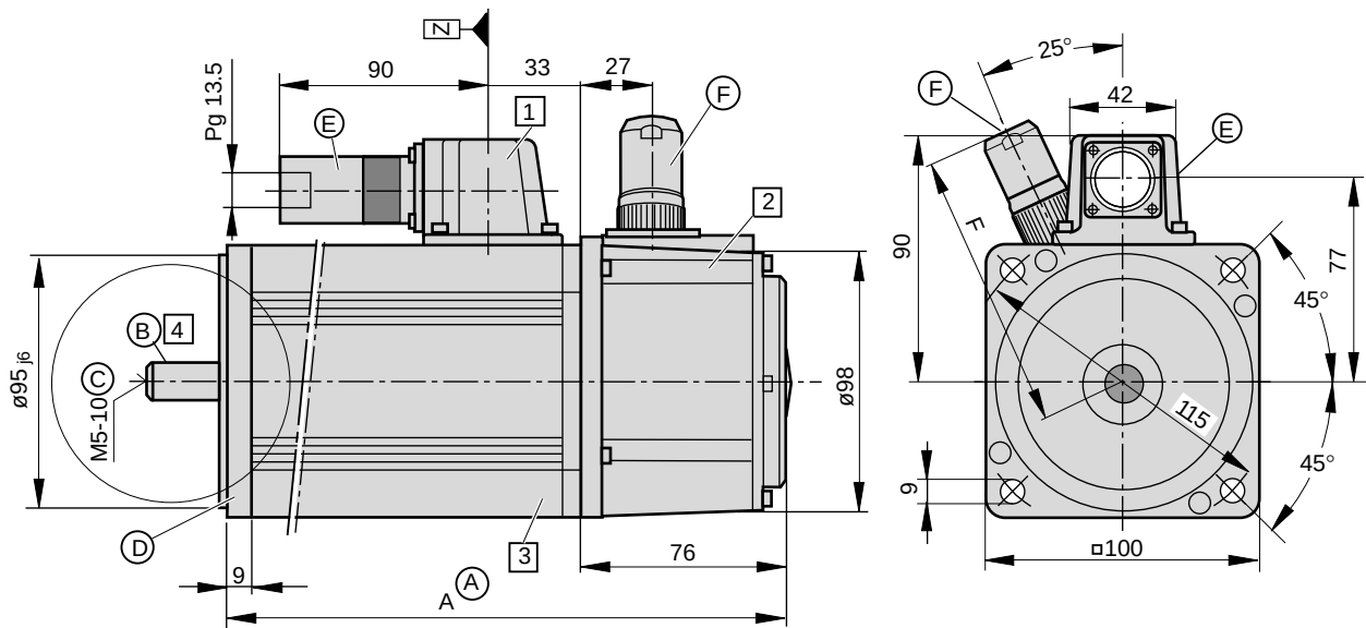
Detail Y
