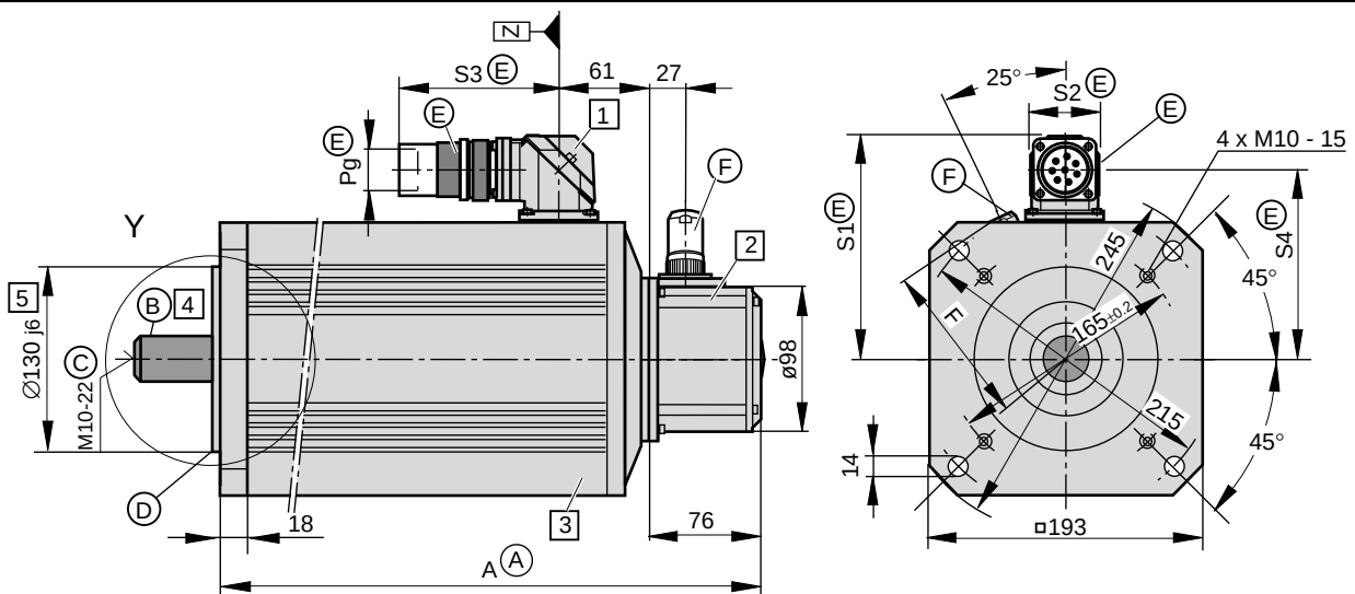
Detail Y
