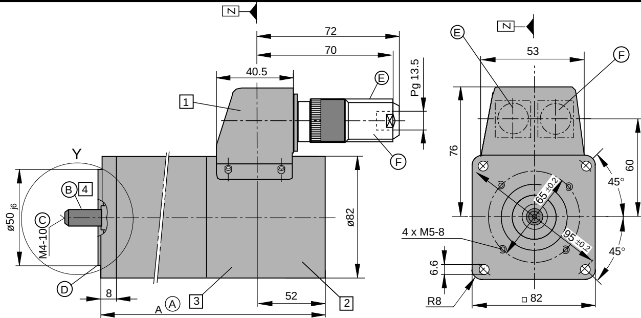
Detail Y
