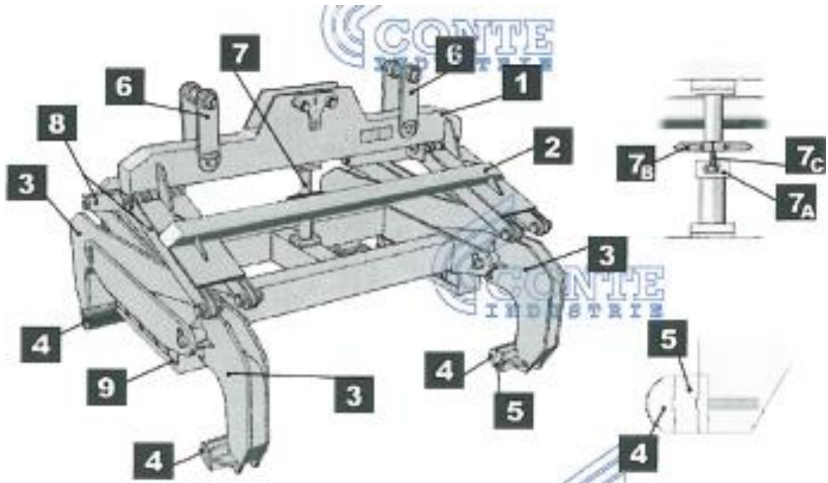
Fig. 1.8.2 Descrizione attrezzatura
