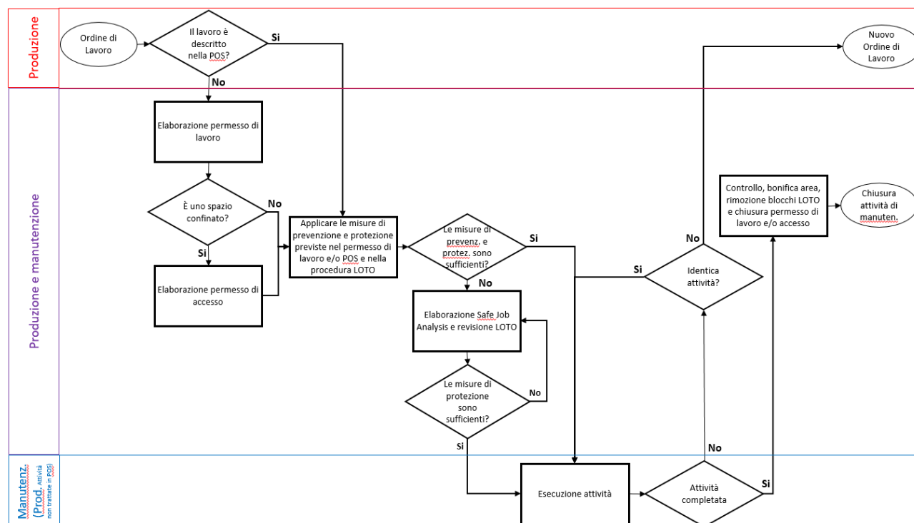
Fig. 2.2-1 – Processo decisionale circa l'emissione dei permessi di lavoro e di accesso
