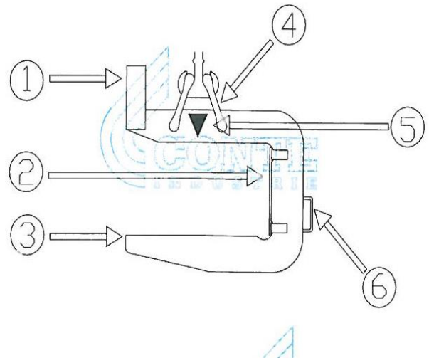
Fig. 3.1-1. Composizione del Gancio a "C"
