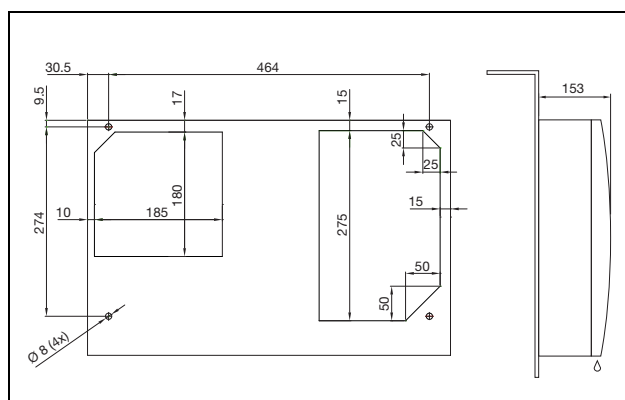
Fig. 92: 3302.3xx sporgente
