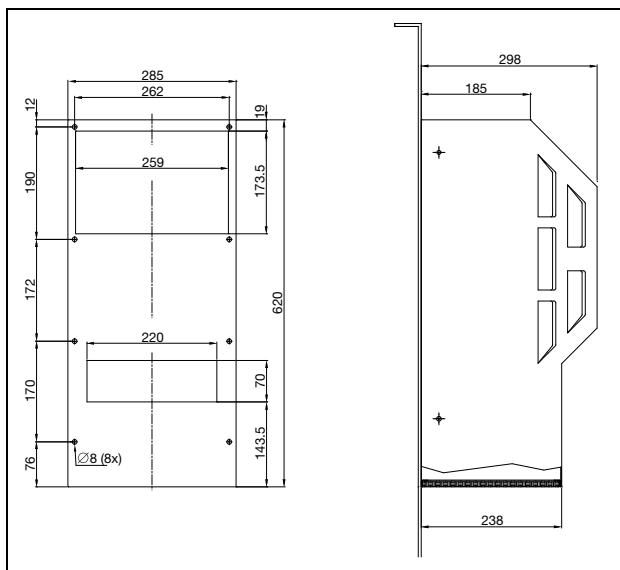
Fig. 98: 3303.xx4
