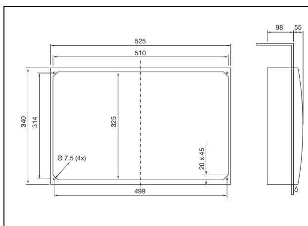
Fig. 106: 3302.3xx incassato
