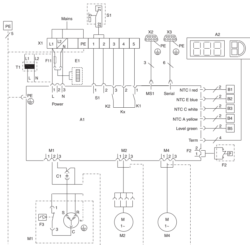
Fig. 114: Schema degli allacciamenti elettrici nr. 4
