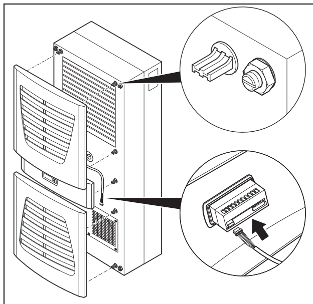
Fig. 27: Collegamento del display e reinserimento della griglia di aerazione
