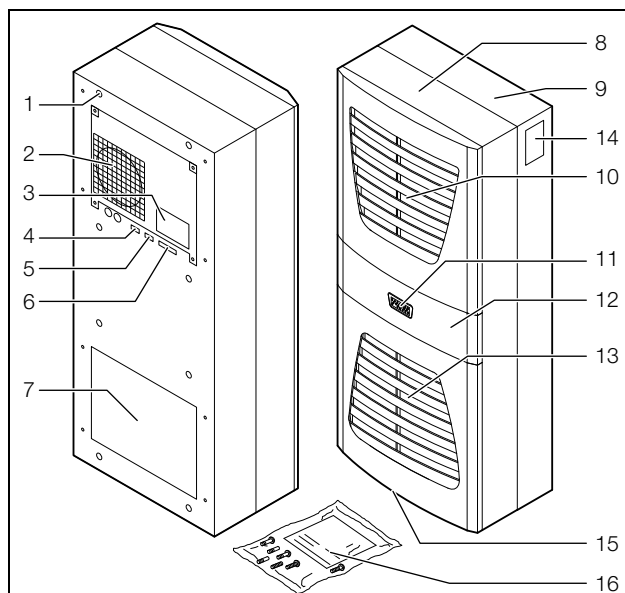
Fig. 2: Descrizione dell'apparecchio
