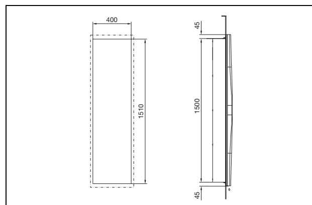
Fig. 110: 3366.xxx incassato
