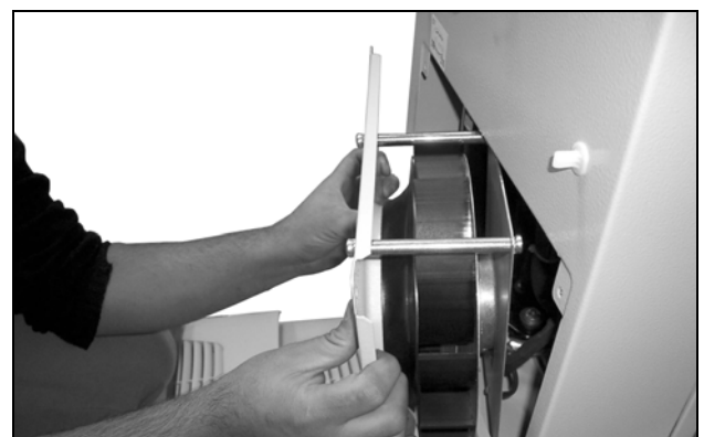
Fig. 42: Smontare il ventilatore
