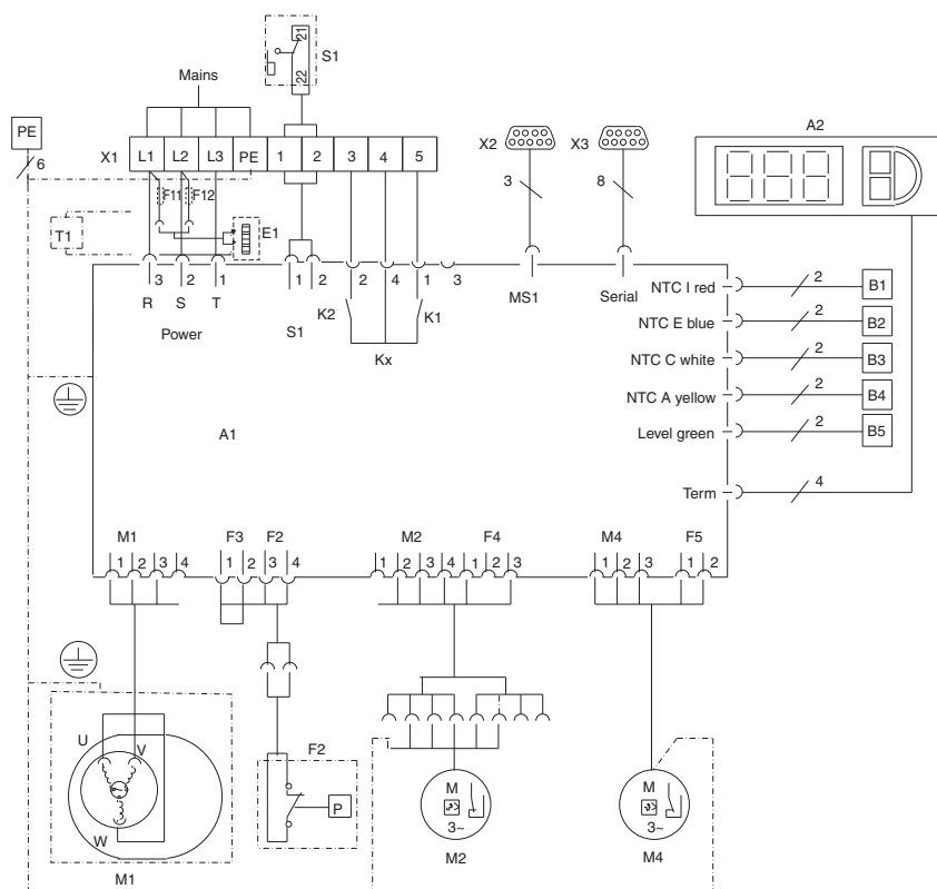
Fig. 118: Schema degli allacciamenti elettrici nr. 8
