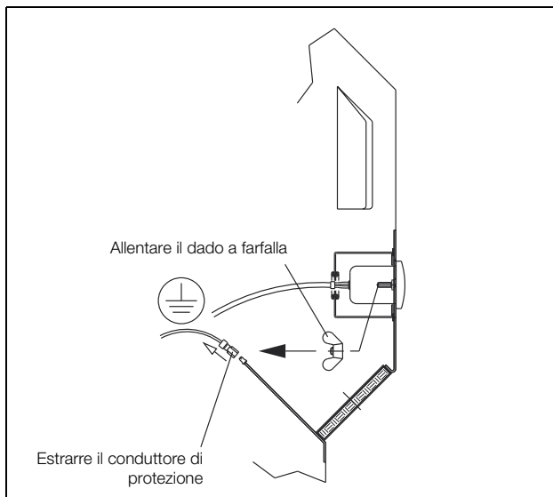
Fig. 80: Smontaggio della cuffia (2)
