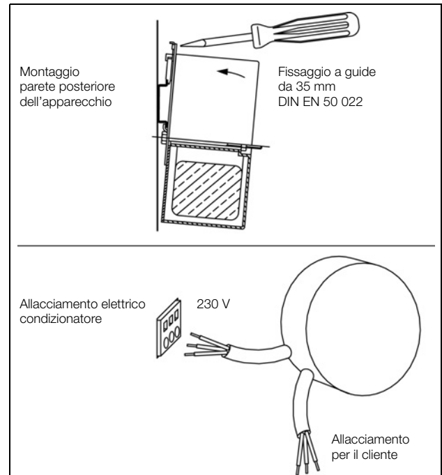
Fig. 20: Montaggio del trasformatore esterno (solo 3361.x40)
