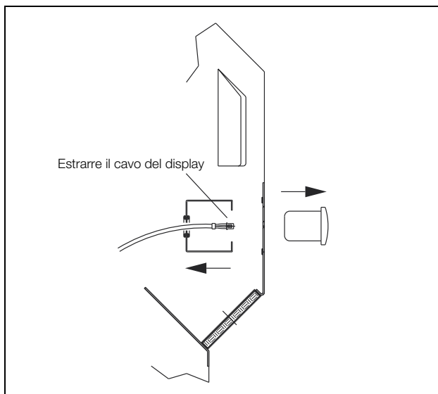
Fig. 81: Smontaggio della cuffia (3)
