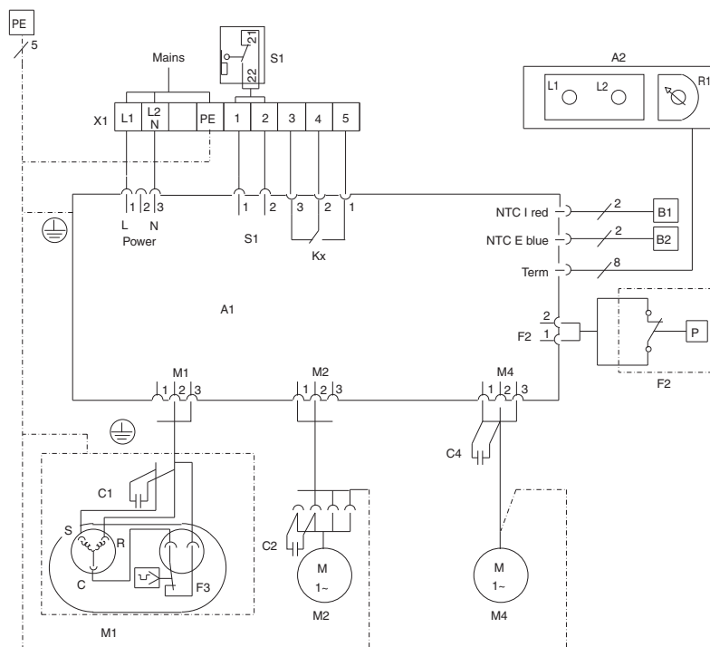
Fig. 111: Schema degli allacciamenti elettrici nr. 1
