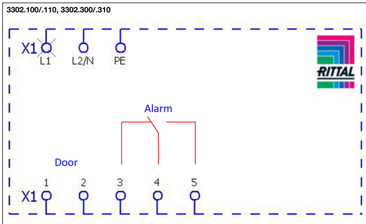
Fig. 23: Schema degli allacciamenti elettrici nr. 1
