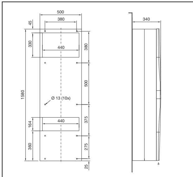
Fig. 97: 3332.xxx sporgente
