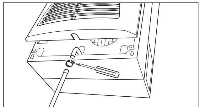
Fig. 19: Collegamento dello scarico di condensa
