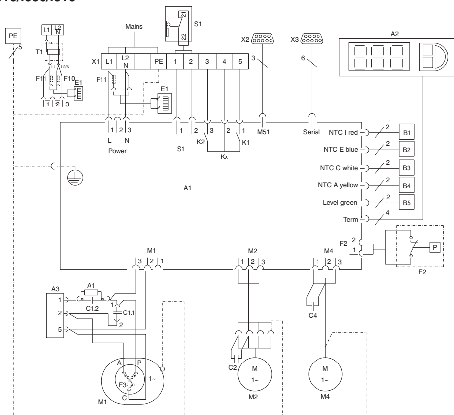
Fig. 117: Schema degli allacciamenti elettrici nr. 7
