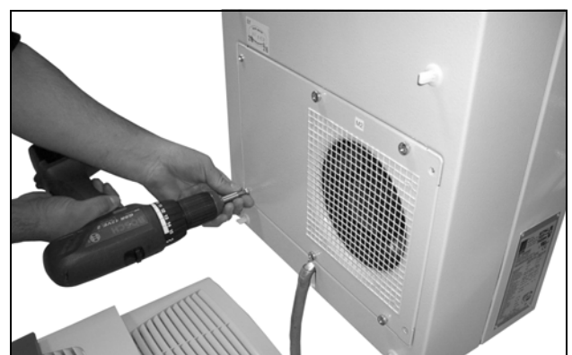
Fig. 41: Smontare il ventilatore del circuito esterno (allentare le quattro viti)
