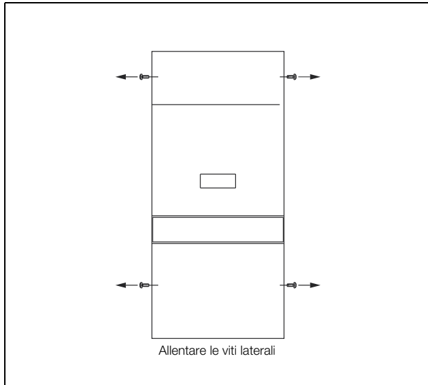
Fig. 79: Smontaggio della cuffia (1)
