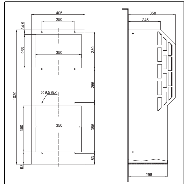
Fig. 99: 3304-5.5x4
