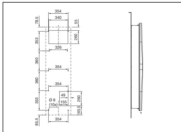
Fig. 94: 3366.xxx sporgente
