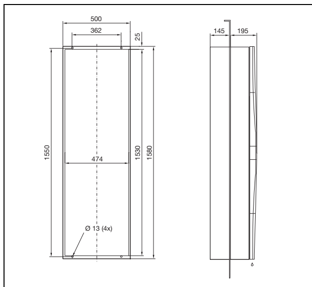
Fig. 104: 3332.xxx semincassato
