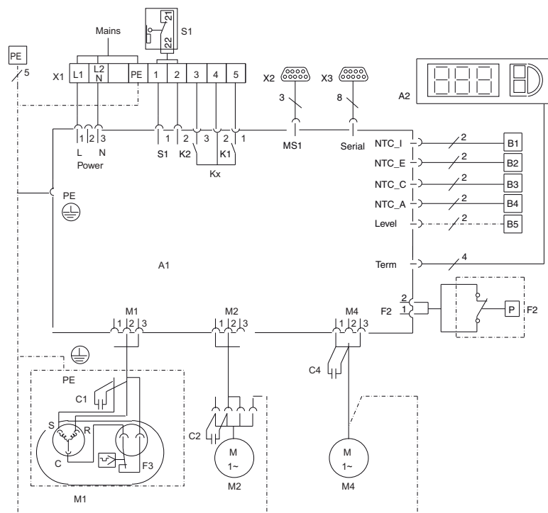
Fig. 112: Schema degli allacciamenti elettrici nr. 2
