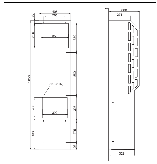
Fig. 100: 3328-29.5x4
