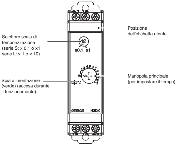
Vista frontale
