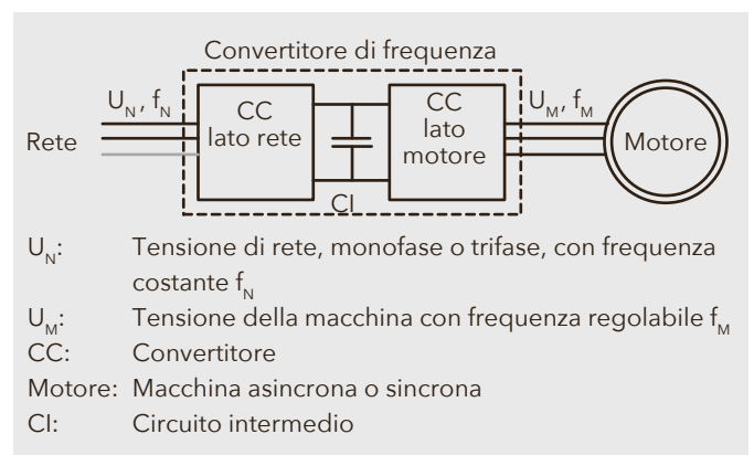
Figura 6: Convertitore di frequenza con circuito intermedio a tensione e motore
