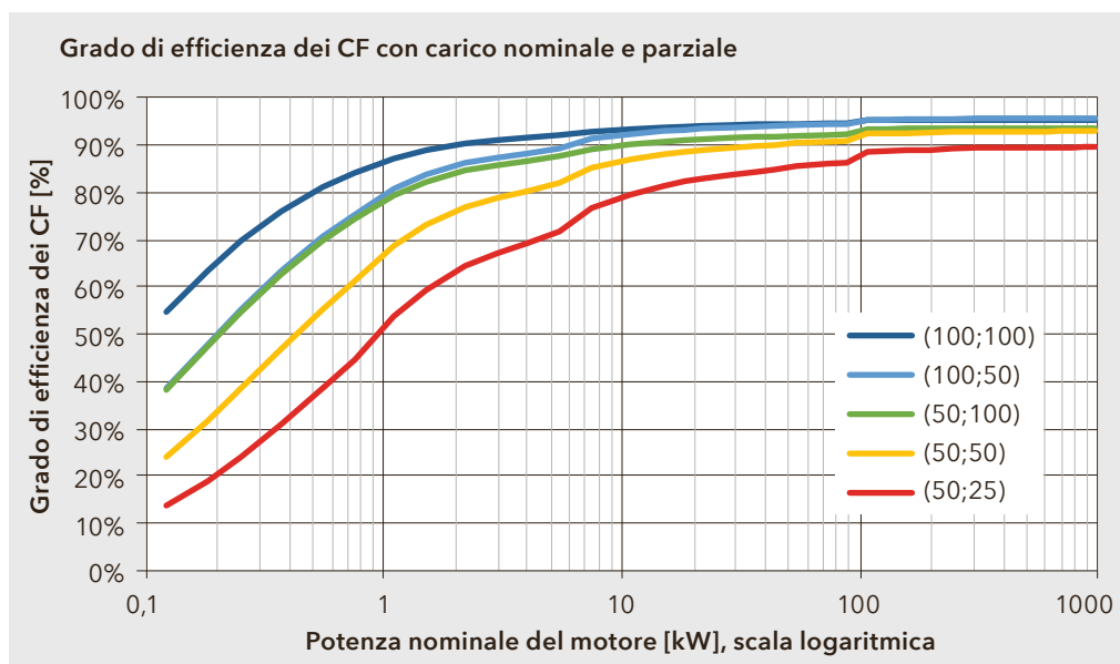
Figura 13: Efficienza del CF in funzione delle dimensioni del motore e del CF con cinque carichi diversi. La figura mostra che a bassa velocità o a bassa coppia, un CF subisce un calo significativo dell'efficienza rispetto all'efficienza alla potenza nominale (fonte: IEC 61800-9-2, ed.1, 2017).
