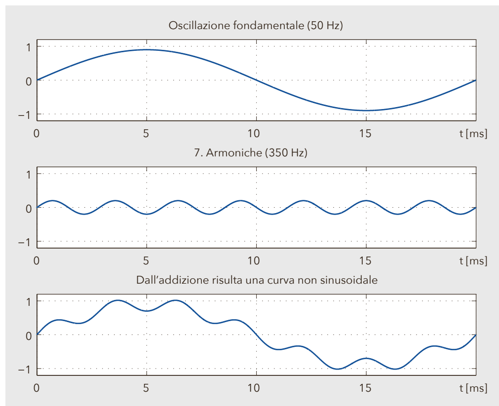
Figura 8: Illustrazione di un segnale (sotto) composto da un'oscillazione fondamentale (sopra) e una settima armonica (al centro).
