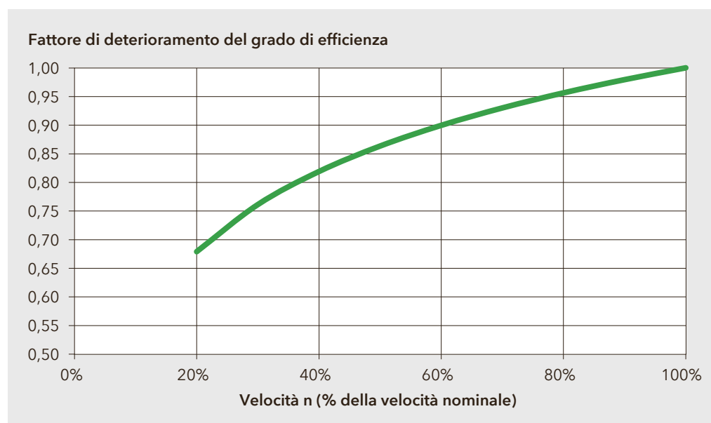
Figura 18: Fattore di deterioramento dell'efficienza del ventilatore e del motore nel funzionamento a carico parziale
