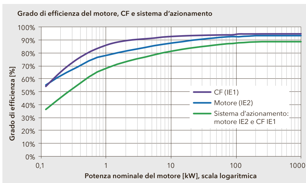
Figura 12: Efficienza del motore, del CF e del sistema di azionamento alla potenza nominale (fonte: IEC 61800-9-2, ed.1, 2017).
