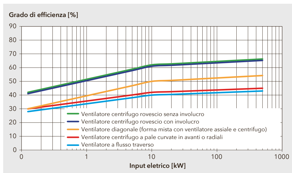
Figura 17: Requisiti di efficienza UE per diversi tipi di ventilatori (2ª fase), rendimento complessivo compreso il motore. Le curve si basano sulla combinazione del ventilatore con un motore IE2.
