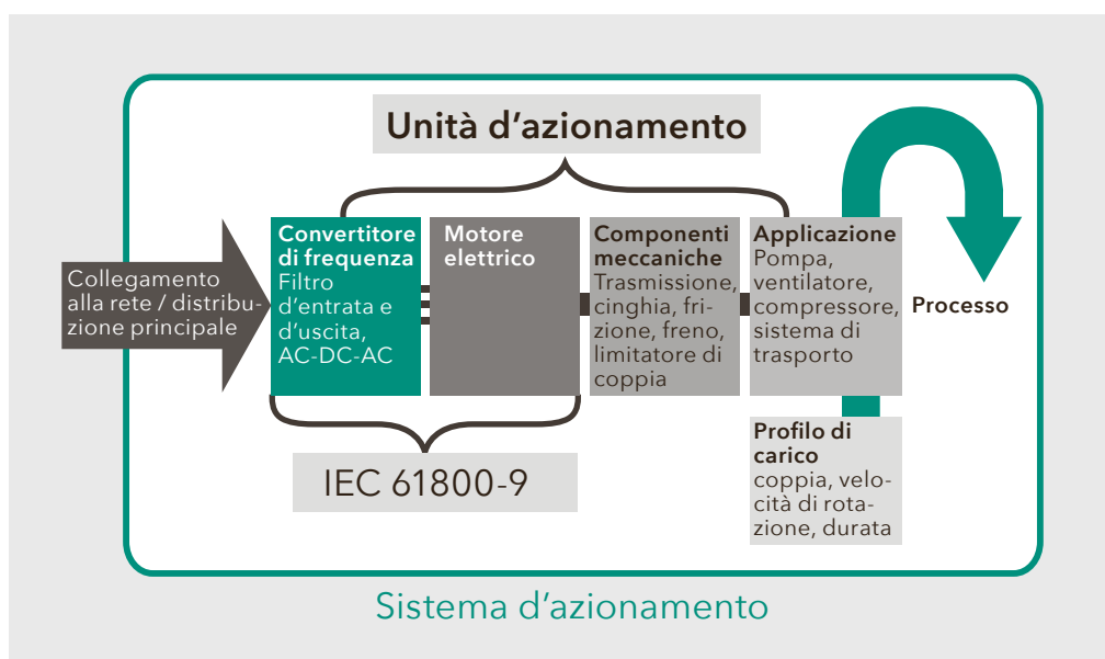
Figura 2: Sistema d'azionamento elettrico. Nella norma IEC 61800-9 sono definiti il metodo di prova e le classi di efficienza dei motori con i CF.
