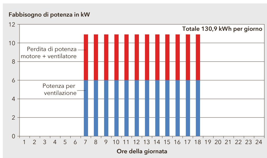
Figura 19: Fabbisogno di potenza elettrica con funzionamento costante senza CF. Totale per l'intera giornata lavorativa = 130,9 kWh (100%)
