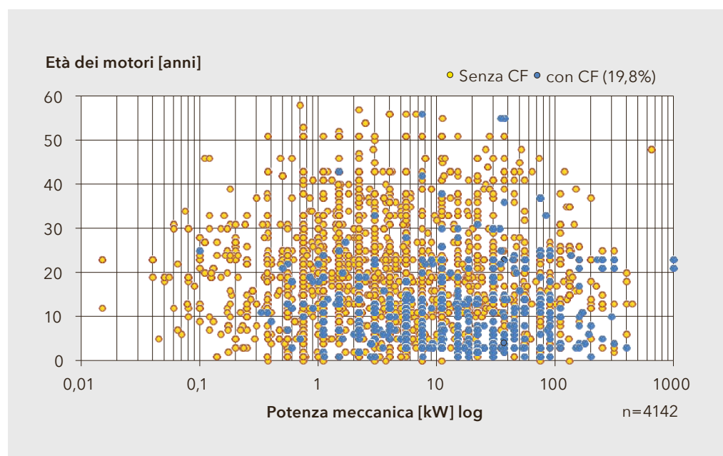
Figura 5: L'analisi di 4142 sistemi d'azionamento ha dimostrato che oggi solo il 19,8% funziona con un convertitore di frequenza (fonte: Easy 2013).
