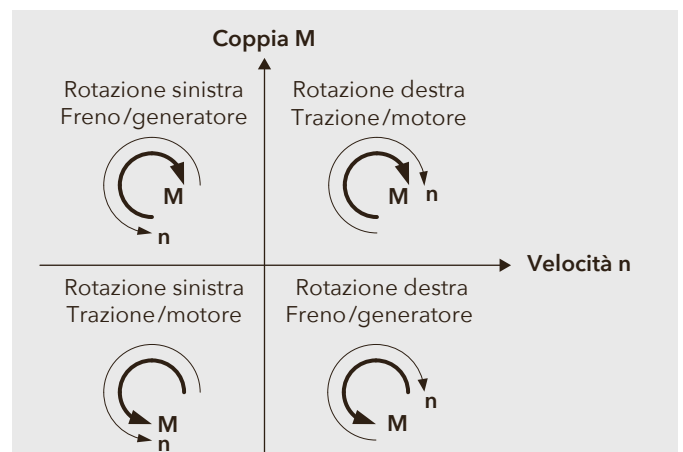
Figura 7: Funzionamento a quattro quadranti di una macchina elettrica
