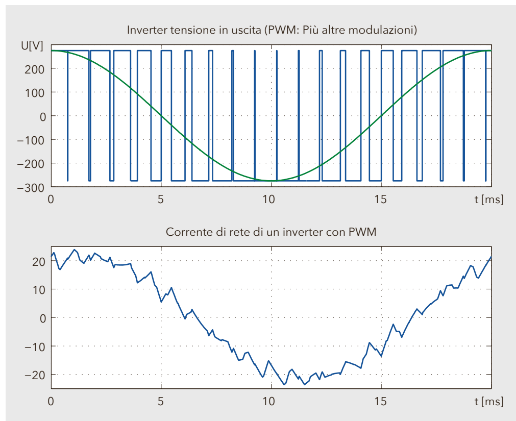
Figura 9: Corso temporale della tensione di uscita dell'inverter di una fase (blu). Modificando l'ampiezza dell'impulso (PWM: modulazione dell'ampiezza dell'impulso) viene simulata nel miglior modo possibile l'oscillazione fondamentale desiderata (verde). Poiché l'inverter può commutare solo avanti e indietro, oltre all'oscillazione fondamentale desiderata si creano delle armoniche. La corrente di fase mostrata nel grafico inferiore è molto più sinusoidale della tensione, ma ha ancora delle armoniche. La frequenza di commutazione in questo esempio è relativamente bassa, 1000 Hz.
