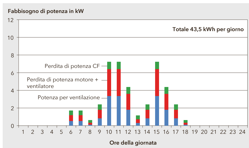
Figura 20: Potenza elettrica richiesta con funzionamento in base al fabbisogno con CF. Totale per l'intera giornata lavorativa = 43,5 kWh (33 %)
