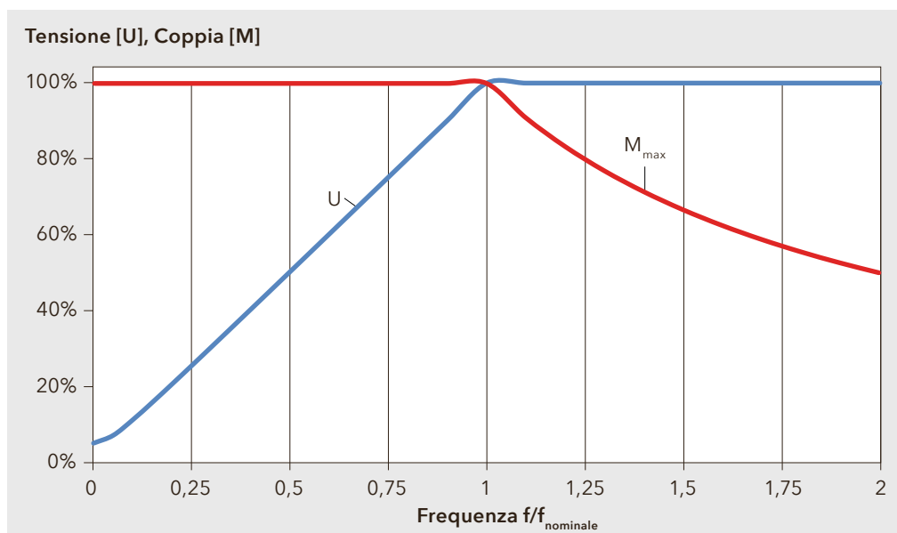
Figura 11: Esempio di curva caratteristica V/f e coppia nominale M
