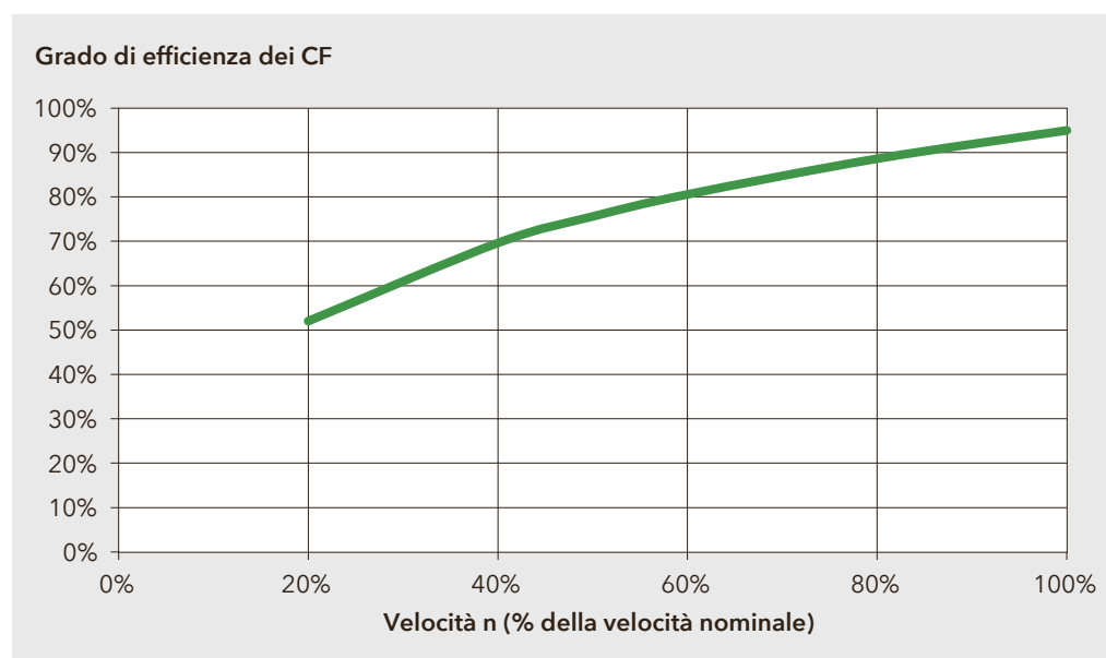
Figura 16: Efficienza del CF per applicazioni con curva di coppia quadratica. Esempio con motore da 11 kW.
