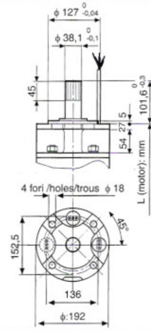
MOTORE/MOTOR/MOTEUR 8" Nema Standard
