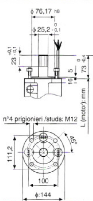
MOTORE/MOTOR/MOTEUR 6" Nema Standard
