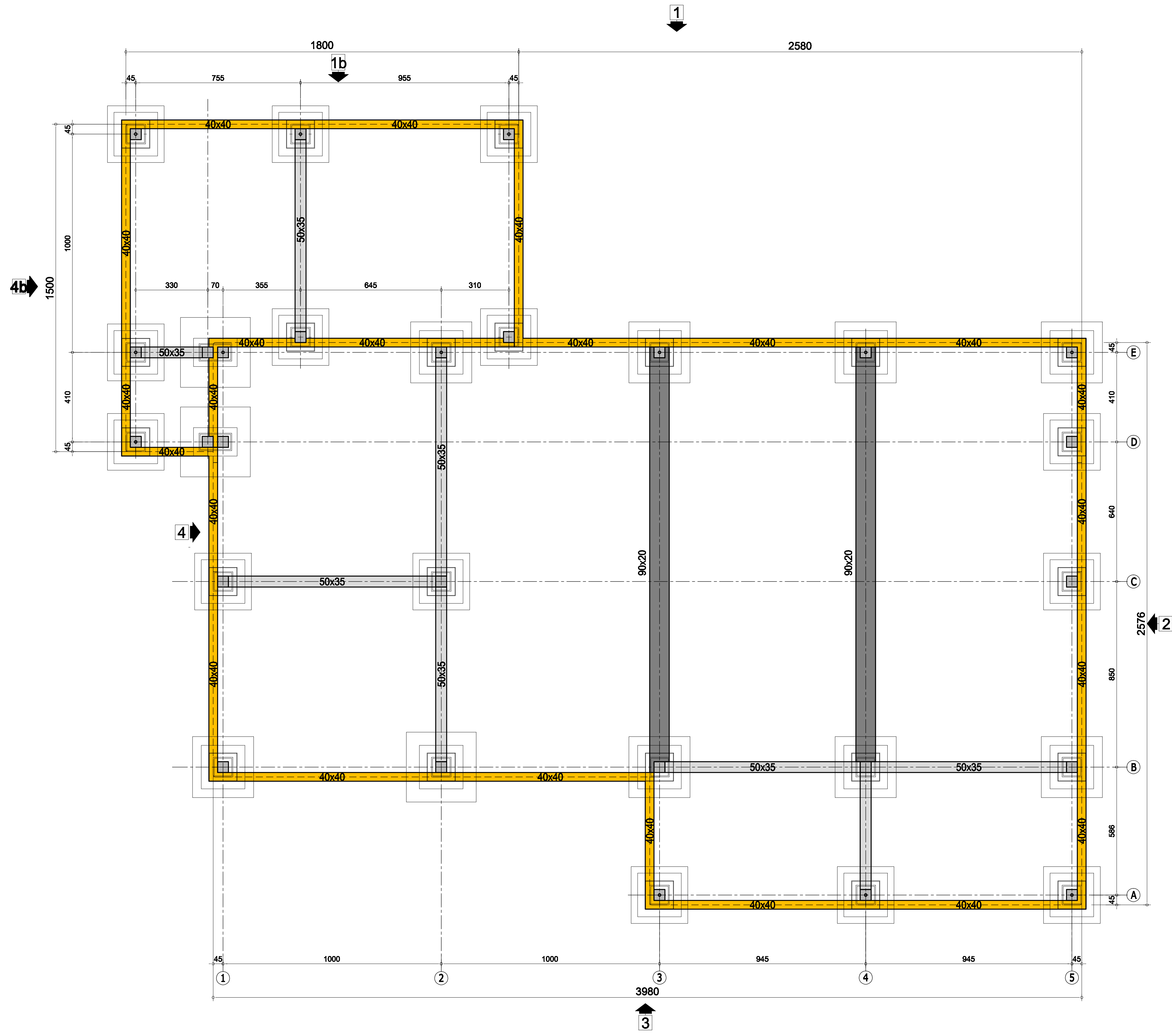
PIANTA FONDAZIONI scala 1:100
