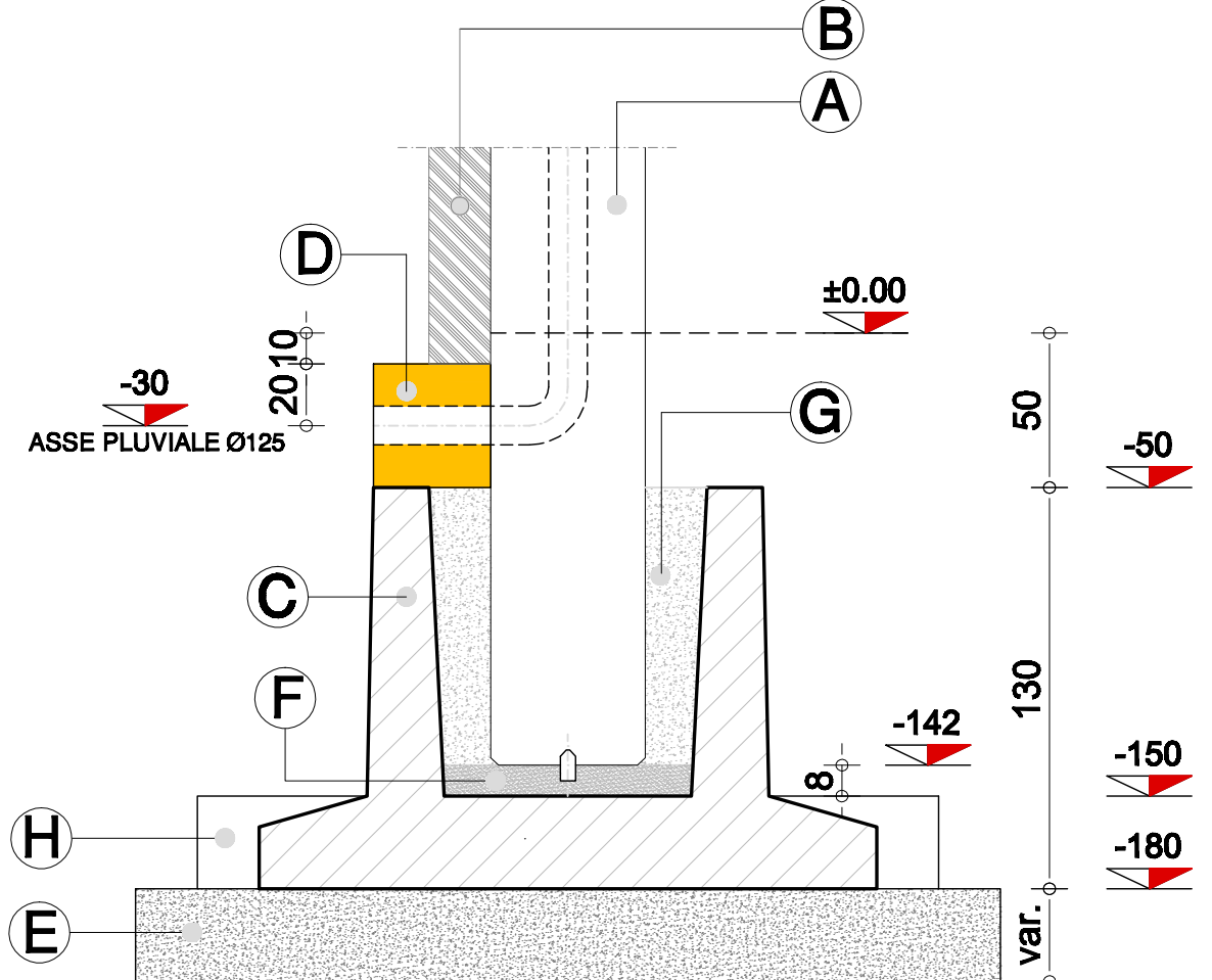
PARTICOLARE FONDAZIONE
