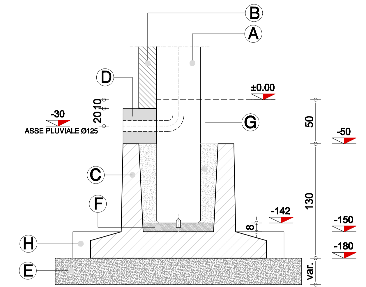
PARTICOLARE FONDAZIONE
