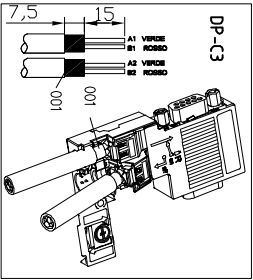
6GK1500-0EA02
