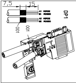
6ES7 972-0BA12-0XA0 90°
