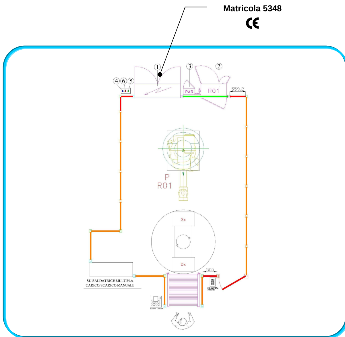
Figura 2 - Lay-Out Isola di saldatura SDPE Bracket DX-SX
