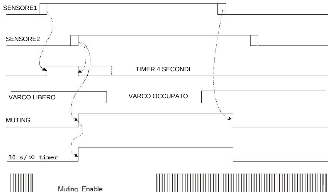
Figura 12 Ciclo di muting
