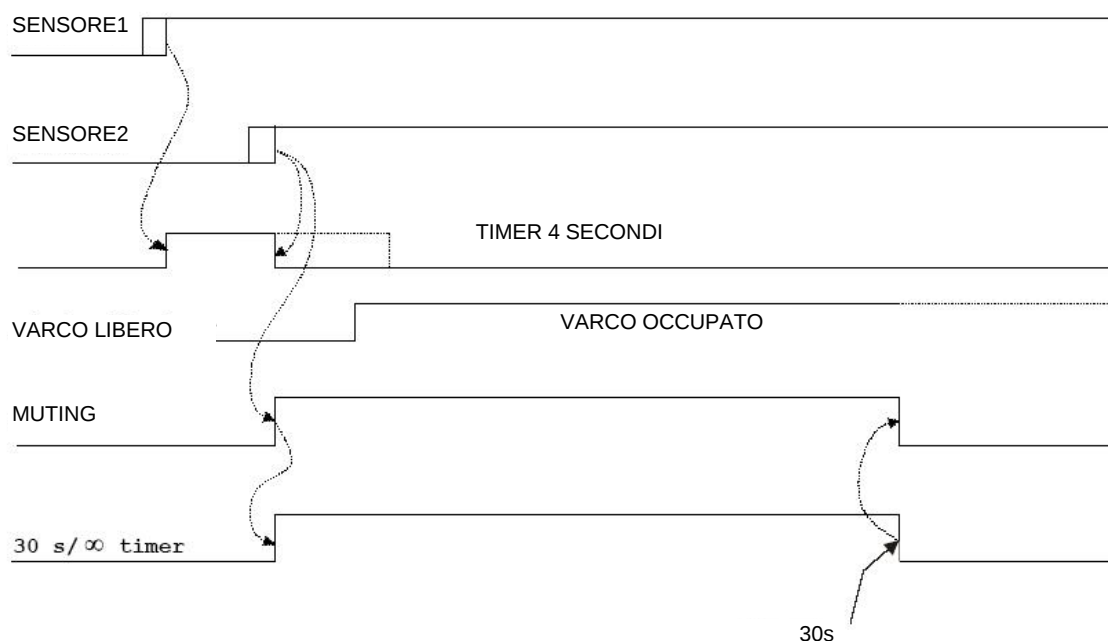
Figura 13 Ciclo di muting che termina grazie ad un timeout
