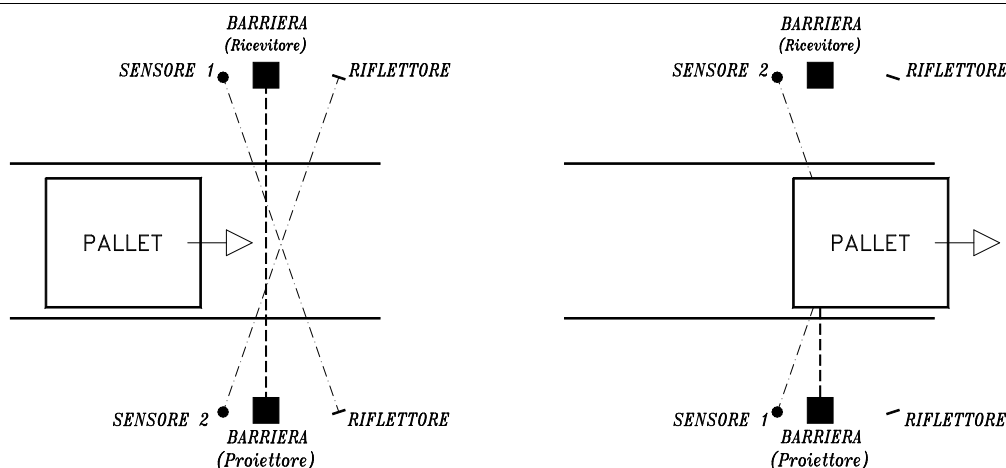
Figura 11 Esempio di applicazione muting su pallettizzatore
