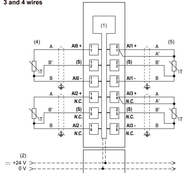
TM5SAI4PH TM5SAI2PH 3 and 4 wires
