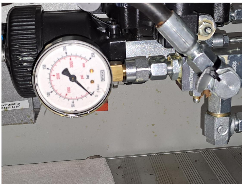
USCITA POMPA DROPSA LUBRIFICAZIONE TESTA T35 - Range: 50-100 bar
