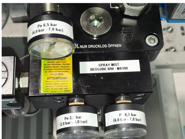
STESSI MANOMETRI, CON DUE FOTO DISTINTE PER VEDERE RANGE, DESCRIZIONE E CAMPO SCALA
