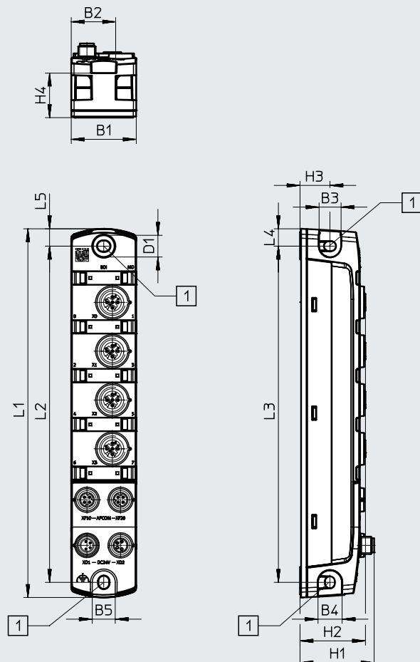
CPX-AP-I-8DI-M12-5P
