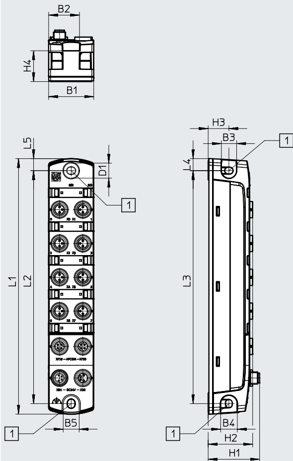
CPX-AP-I-8DI-M8-3P
