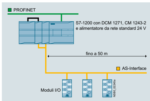
Realizzazione di una rete AS-i Power24V con modulo di disaccoppiamento dati AS-Interface DCM 1271
