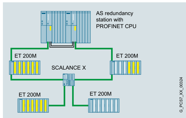
PCS 7 Comunicazione PROFINET IO fail-safe con ridondanza di sistema
