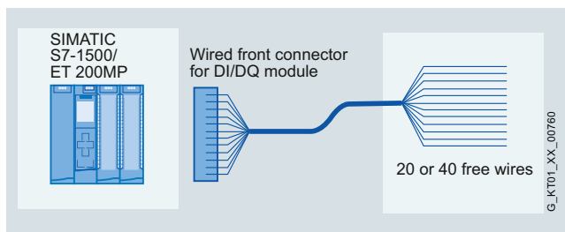
SIMATIC TOP connect per S7-1500/ ET 200MP, collegamento flessibile
