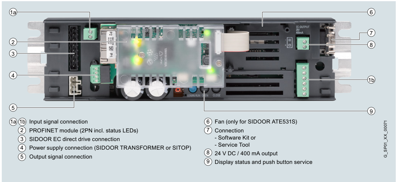
Schema di collegamento SIDOOR ATE530S/531S
