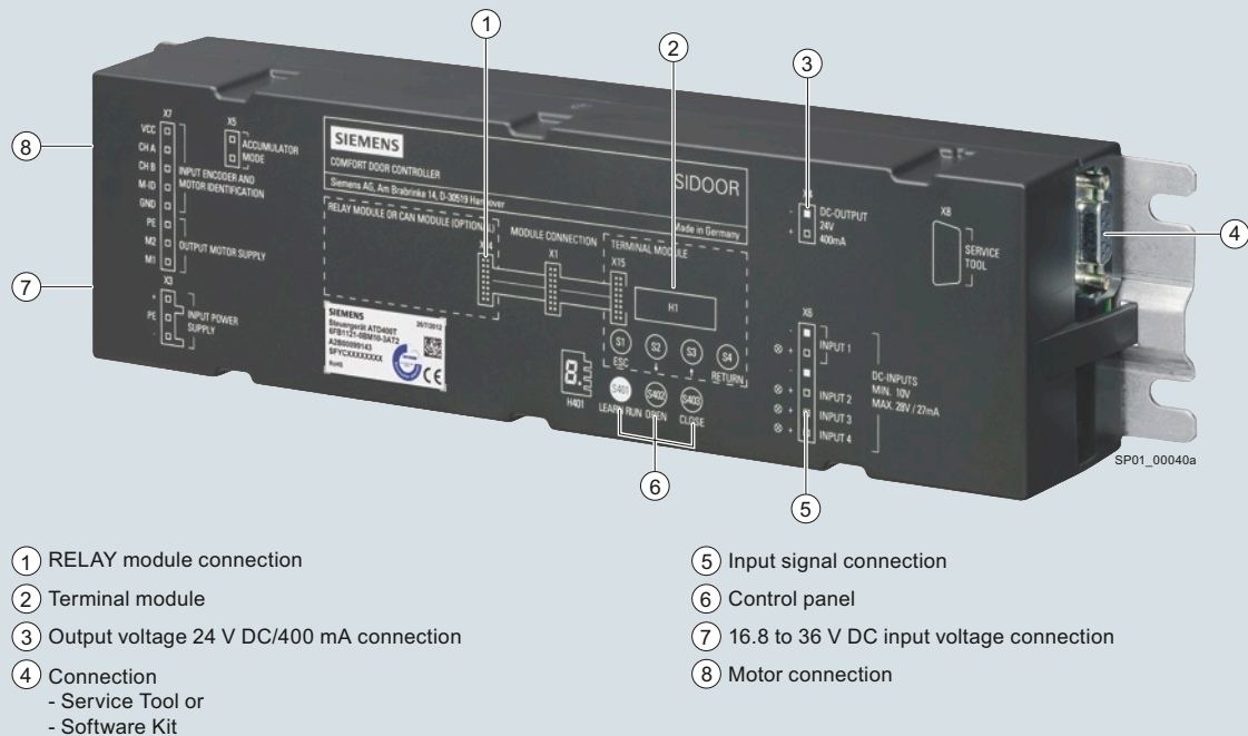
Azionamento per porte interne di treni SIDOOR ATD400T
