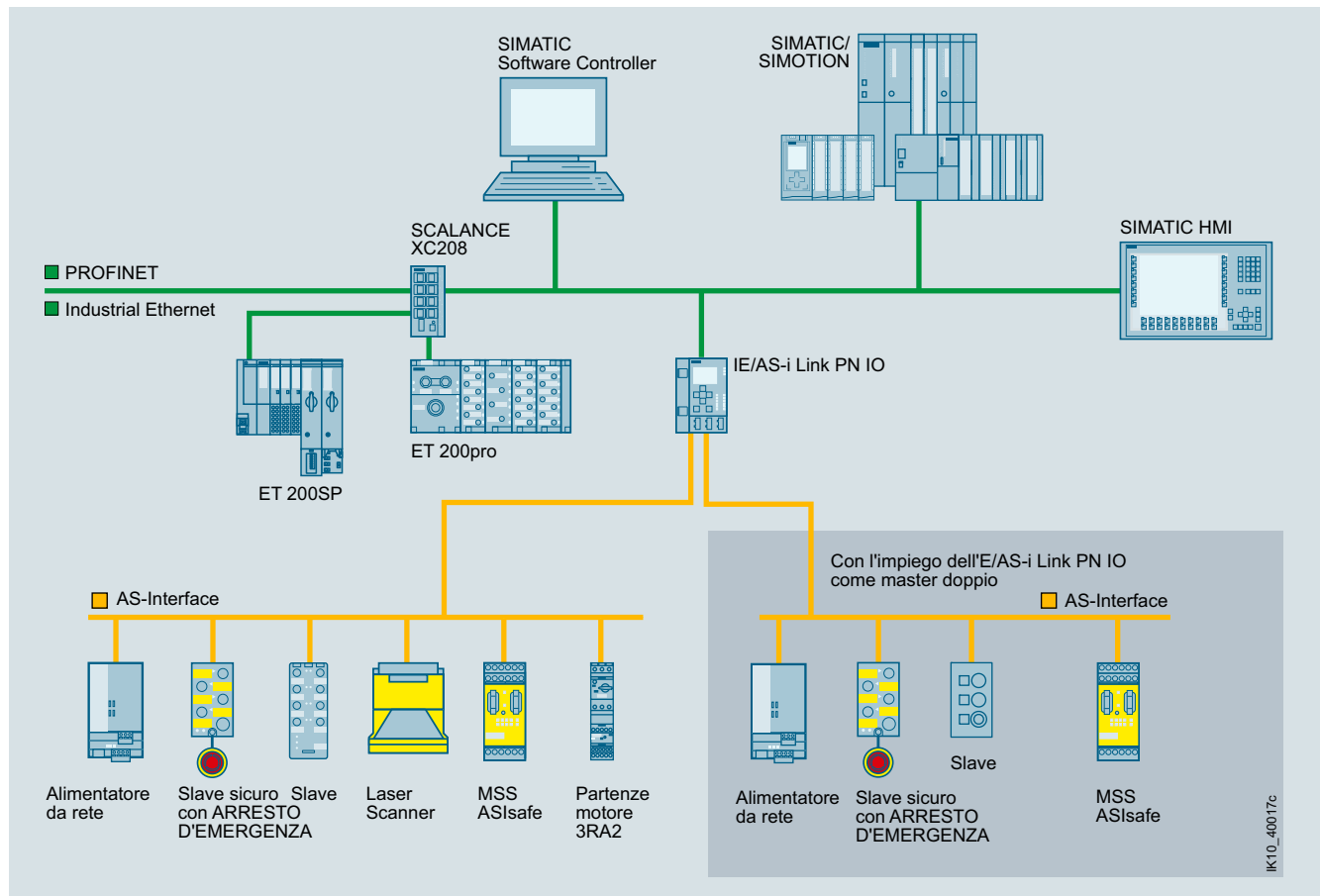
Collegamento di AS-Interface a PROFINET tramite IE/AS-i Link PN IO come master semplice/doppio
