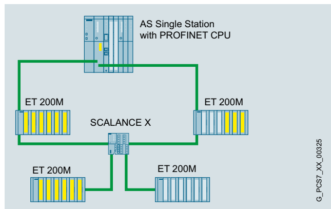
PCS 7 Comunicazione PROFINET IO fail-safe con ridondanza dei mezzi trasmissivi
