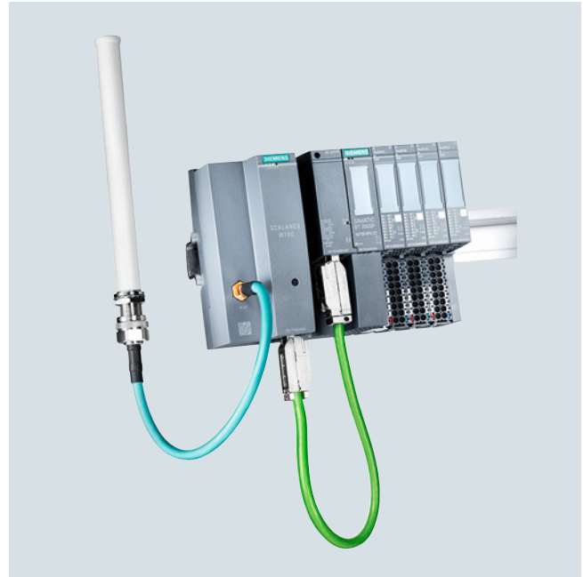
Stazione ET 200MP con SCALANCE W722 RJ45
