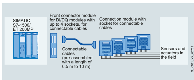
SIMATIC TOP connect per S7-1500/ ET 200MP, collegamento completamente modulare
