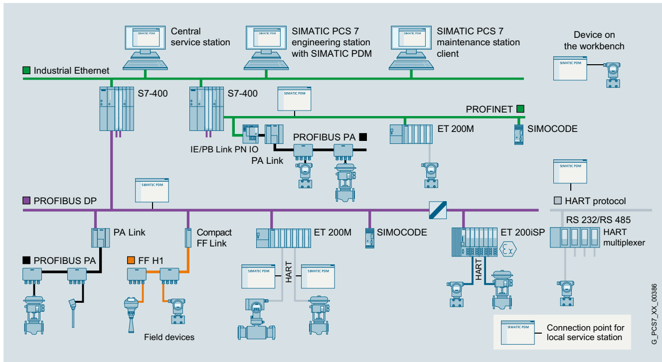
Possibilità di configurazione con SIMATIC PDM
