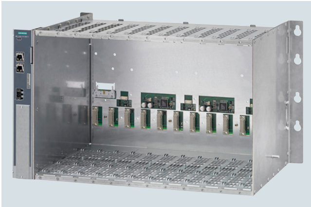
Sistema per controllori di riscaldamento SIPLUS HCS4200
