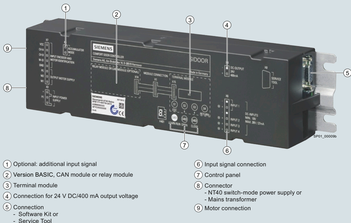
Azionamento porta ascensore SIDOOR AT40 (esecuzione modulo relè)
