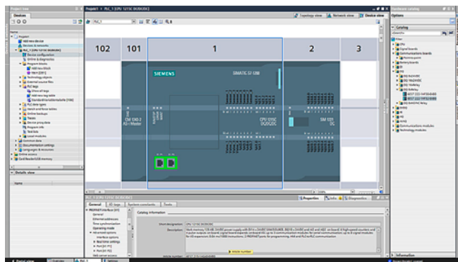
STEP 7 Basic V15.1 (TIA Portal), vista dispositivi: configurazione e parametrizzazione in una rappresentazione fotorealistica
