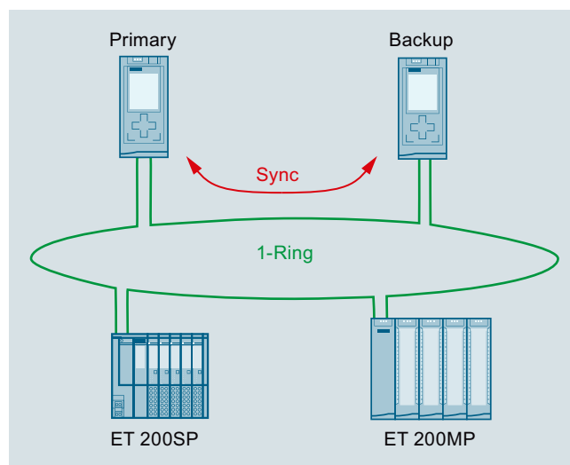
Funzionamento del SIMATIC S7-1500R
