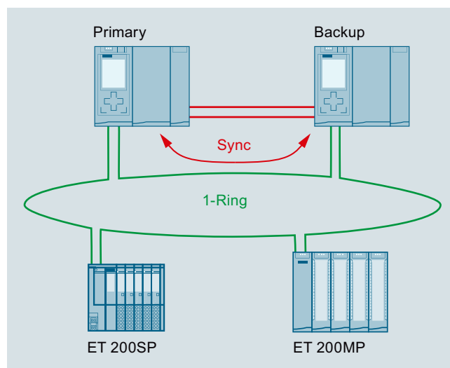
Funzionamento del SIMATIC S7-1500H
