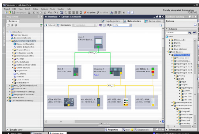
Configurazione di una rete AS-Interface con CM AS-i Master ST tramite il TIA Portal
