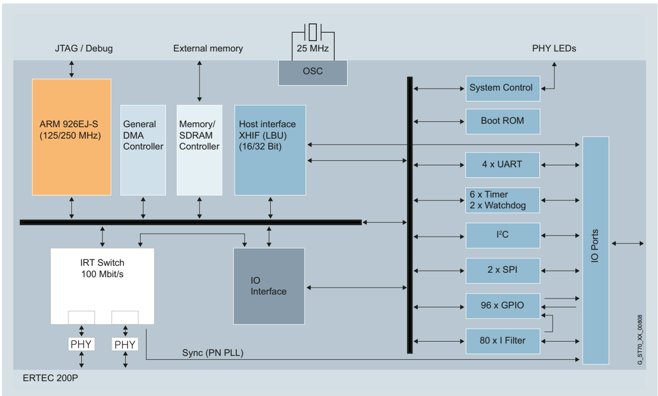
Struttura interna di ERTEC 200P-2
