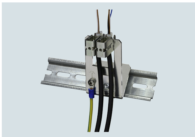
Supporto per schermi 6AT8002-4AA00
