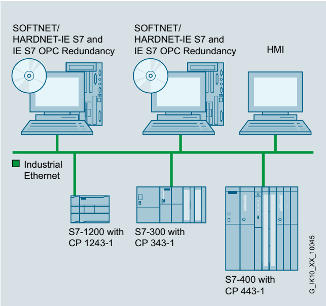
Configurazione di sistema SOFTNET per Industrial Ethernet
