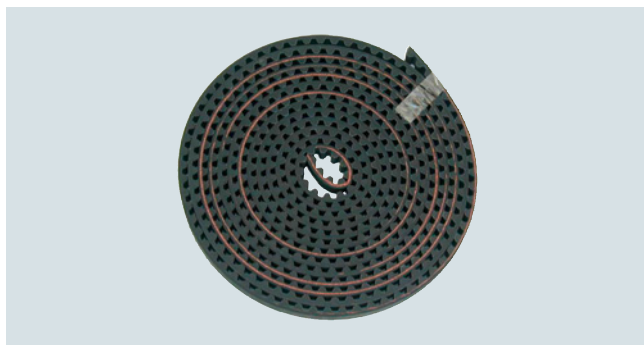
Cinghia dentata 6FB1104-0AT01-0AB0 (larghezza 12 mm, lunghezza 4 m)
