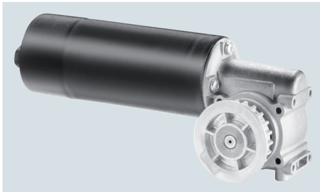
Motoriduttore EC SIDOOR MEG251 L, 6FB1203-5AT00-7MP0. (Esecuzione con pignone a sinistra)
