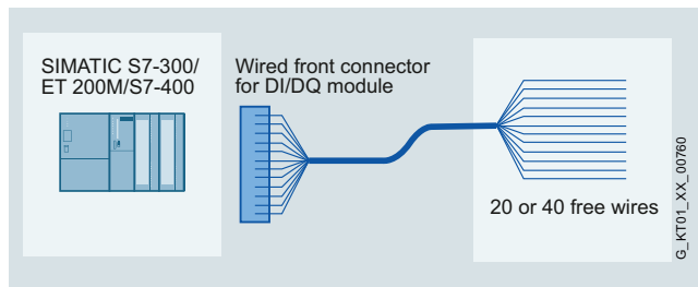
SIMATIC TOP connect per S7-300/ET200M, collegamento flessibile
